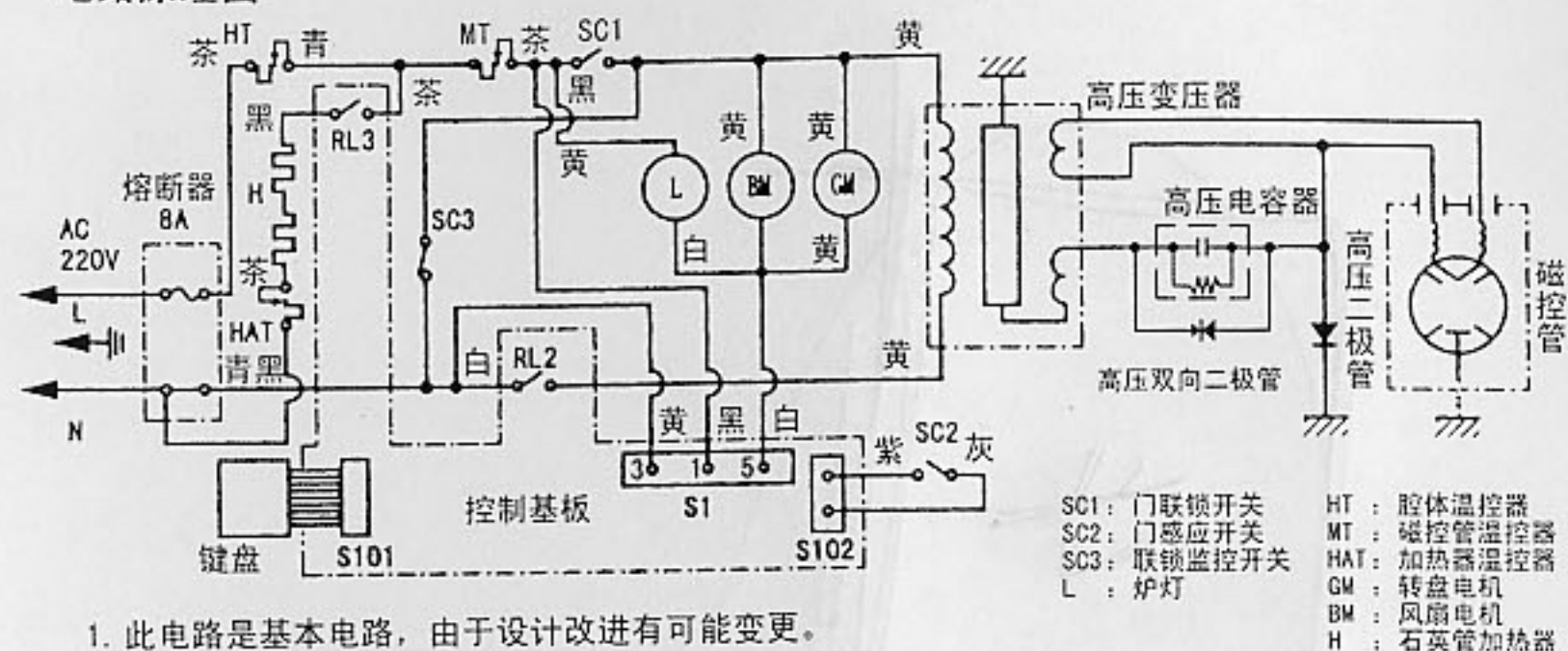
电路原理图
