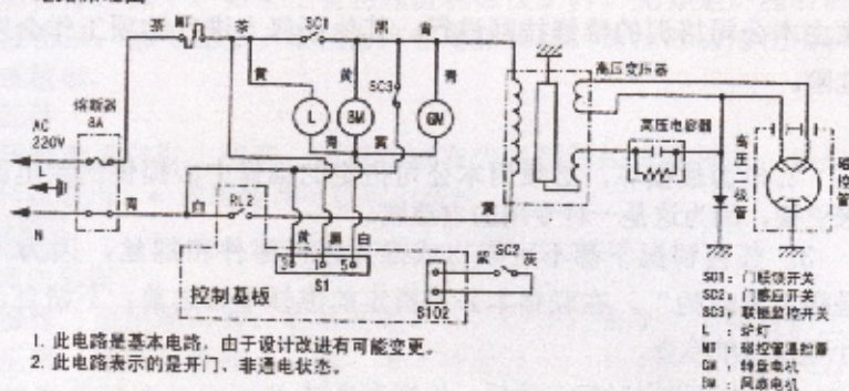
电路原理图
