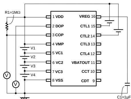
测定电路6
