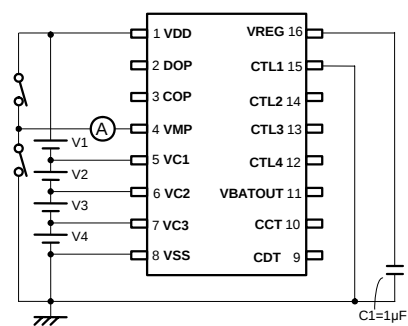
测定电路8
