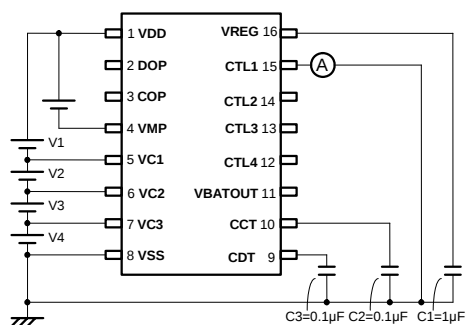
测定电路5
