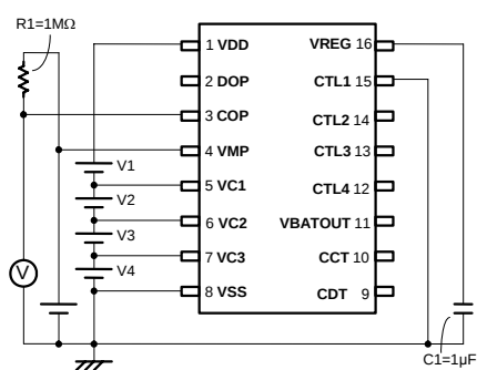
测定电路7
