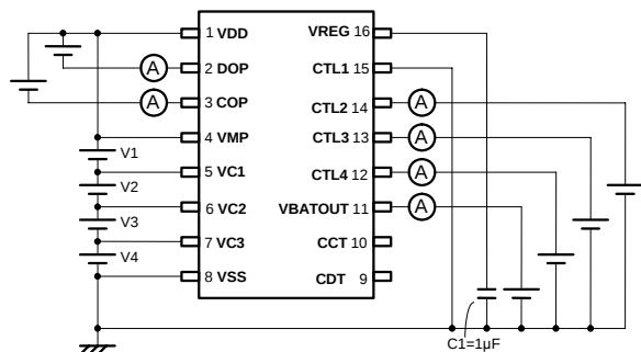
测定电路9
