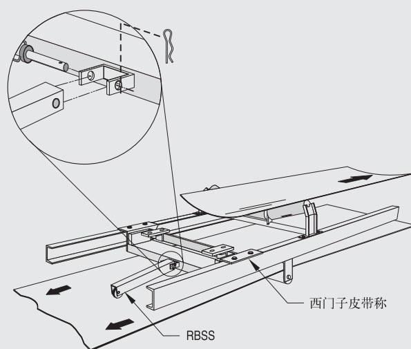
RBSS 安装
