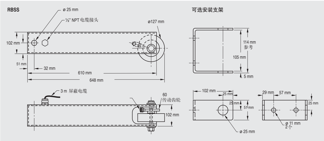
RBSS 尺寸
