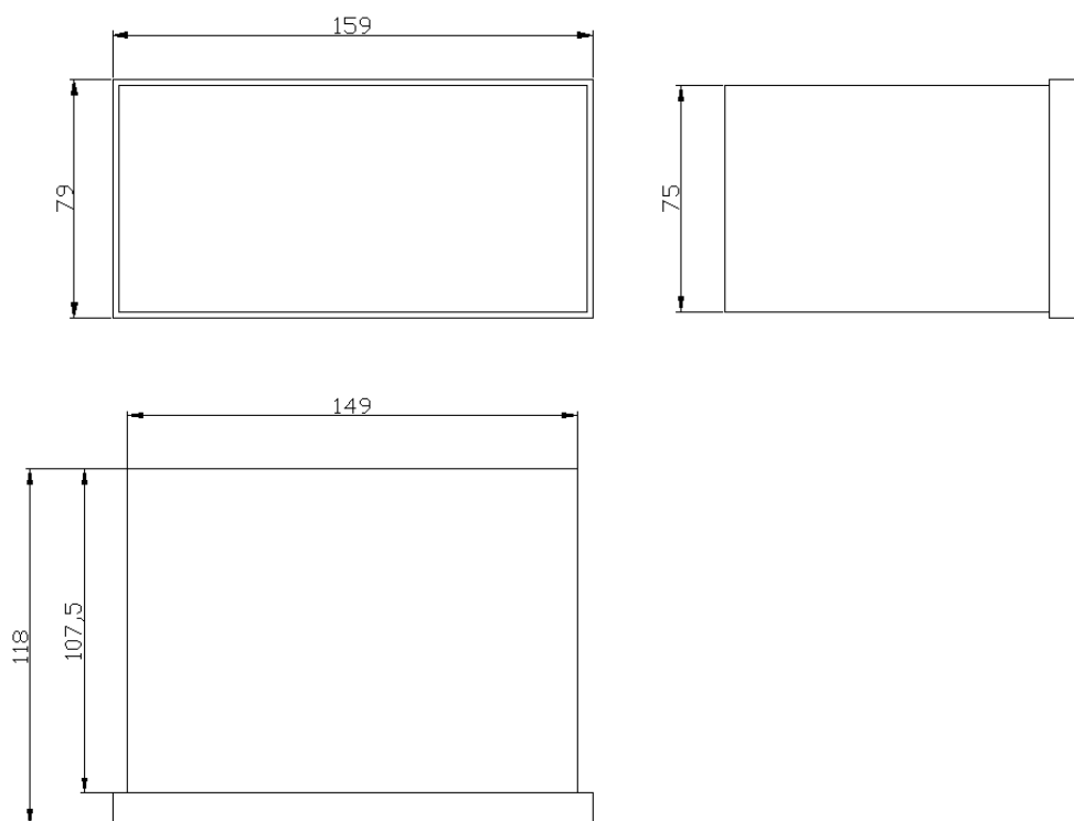
图 1-3 外形尺寸图
