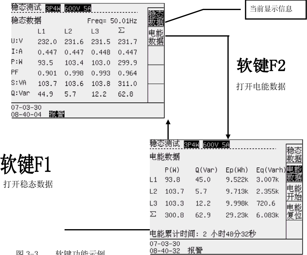
图 3-3 软键功能示例
