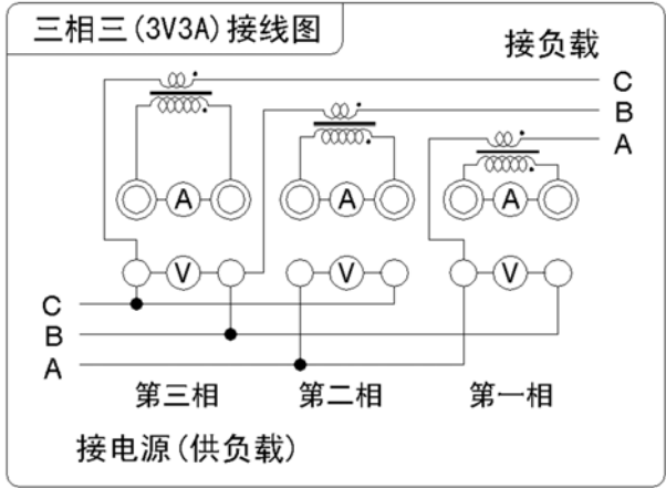
图 4-8 三相三线（3V3A—CT）接线图
