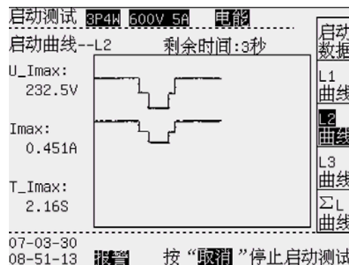
图 11-2 L2 曲线
