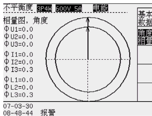
图 8-2 相量角度
