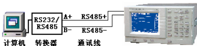
图 14-1 测试仪与计算机通讯—RS485
