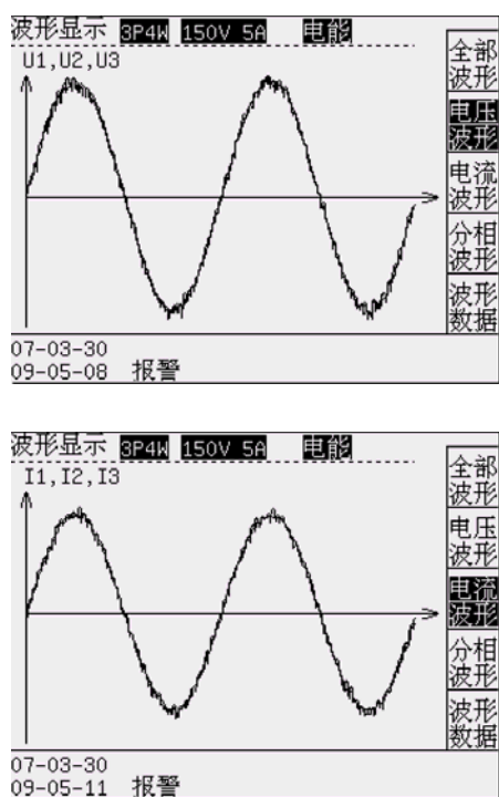
图 6-2 电压波形与电流波形
