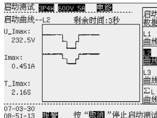
图 10-2 L2 曲线
