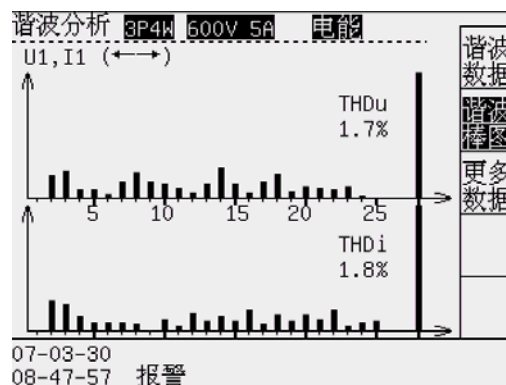
图 7-2 谐波棒图
