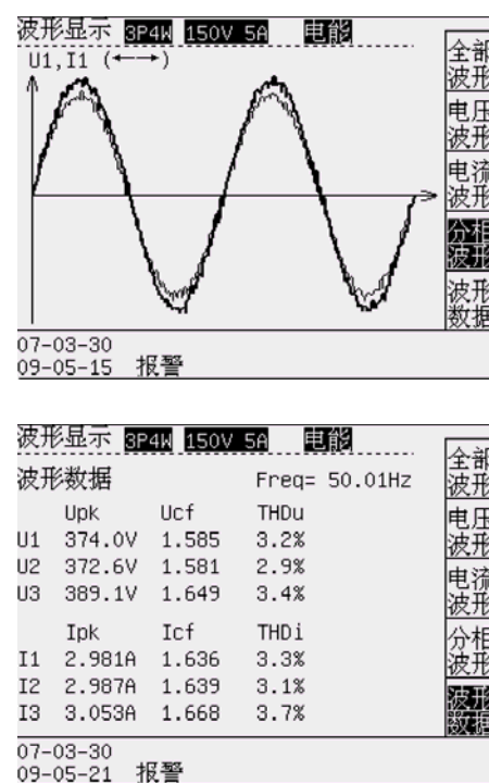
图 6-3 分相波形与波形数据
