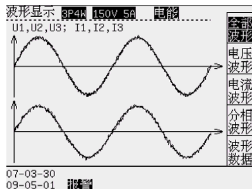
图 6-1 波形显示
