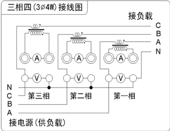
图 4-7 三相四线（3P4W—CT）接线图
