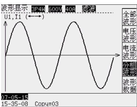
图 2-2 滤波后的变频器输出的电压波形
