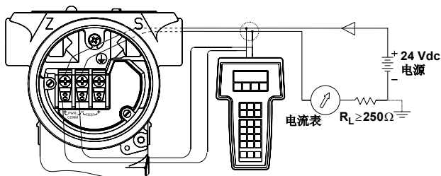
图 3. 低功耗变送器接线图
