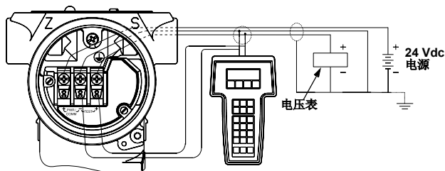
图 3. 低功耗变送器接线图
