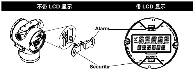
图 1. 变送器的电子线路板
