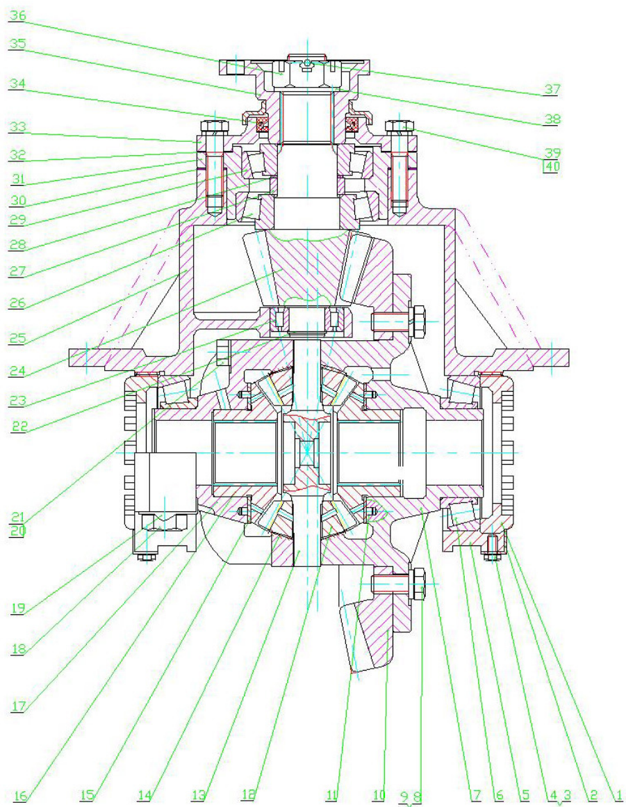
圖三 PR60·21·1結構圖
