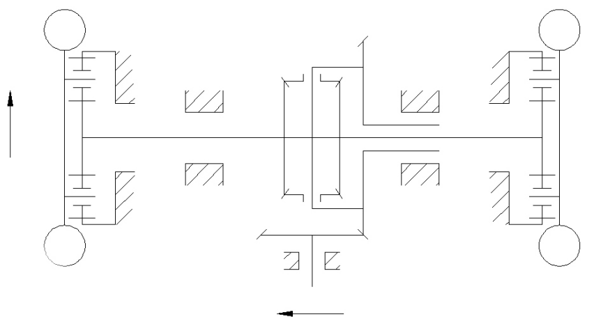
图一 工作原理图
