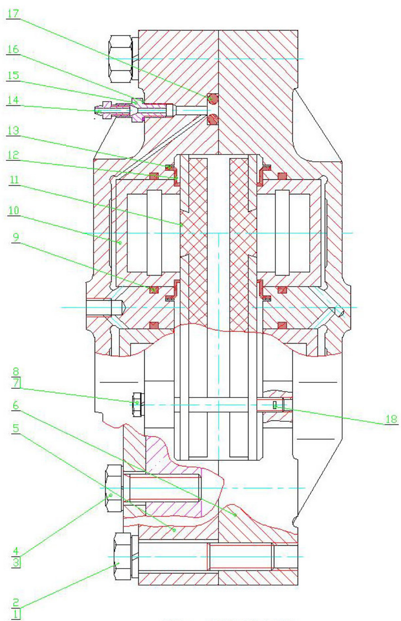
图四 盘式制动器结构图
