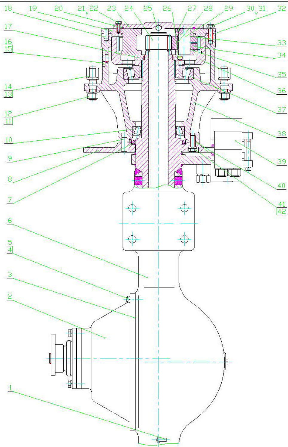
图二 PR60·21B-00 结构图
