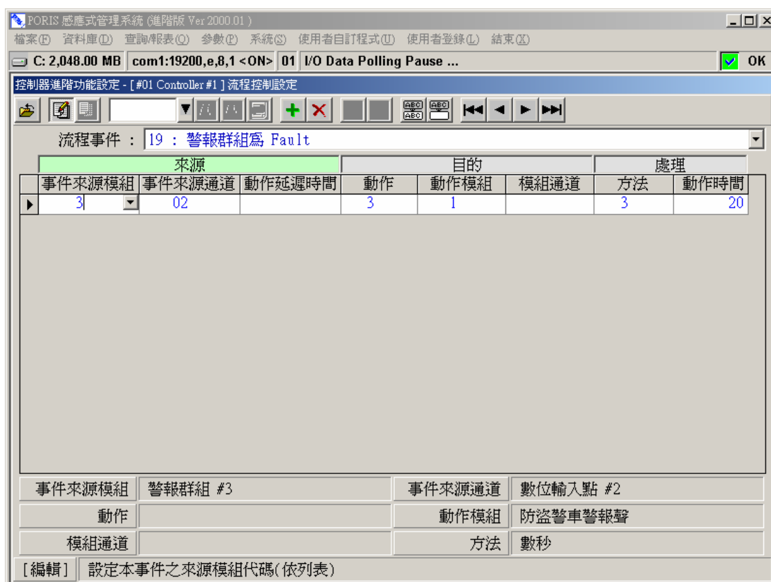
圖 2-19 流程事件 – 警報群組為 Fault
