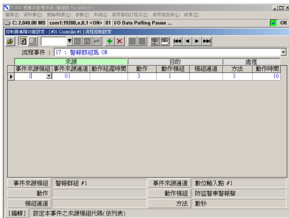
圖 2-17 流程事件 – 警報群組為 ON
