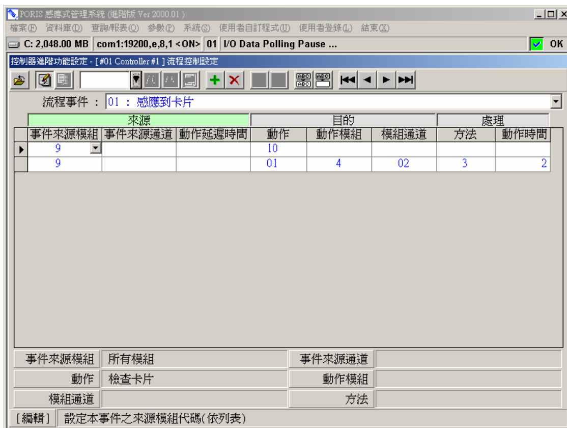
圖 2-1 流程事件 – 感應到卡片
