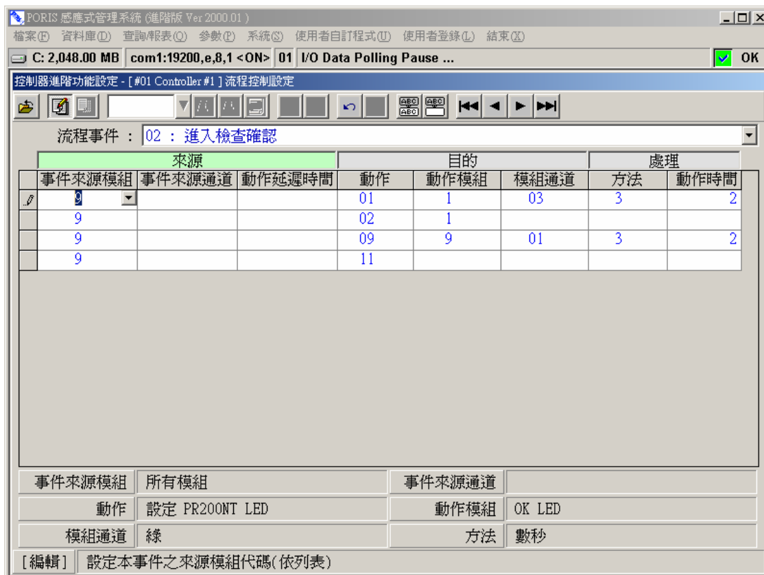
圖 2-2 流程事件 – 進入檢查確認
