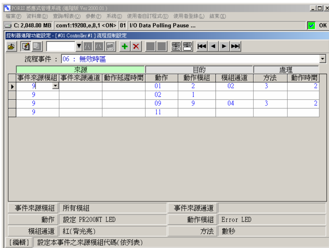
圖 2-6 流程事件 – 無效時區
