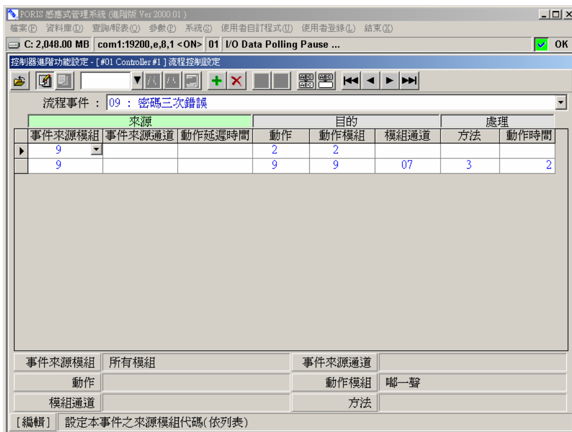
圖 2-9 流程事件 – 密碼三次錯誤
