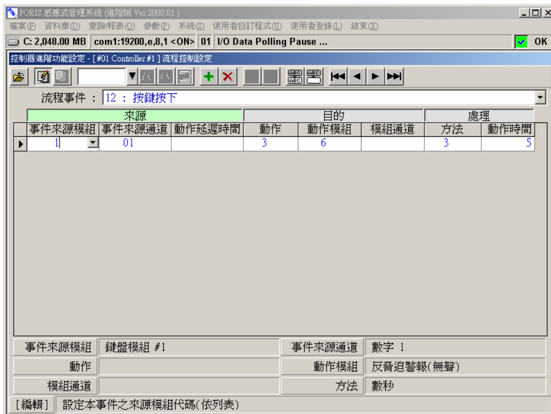
圖 2-12 流程事件 – 按鍵按下
