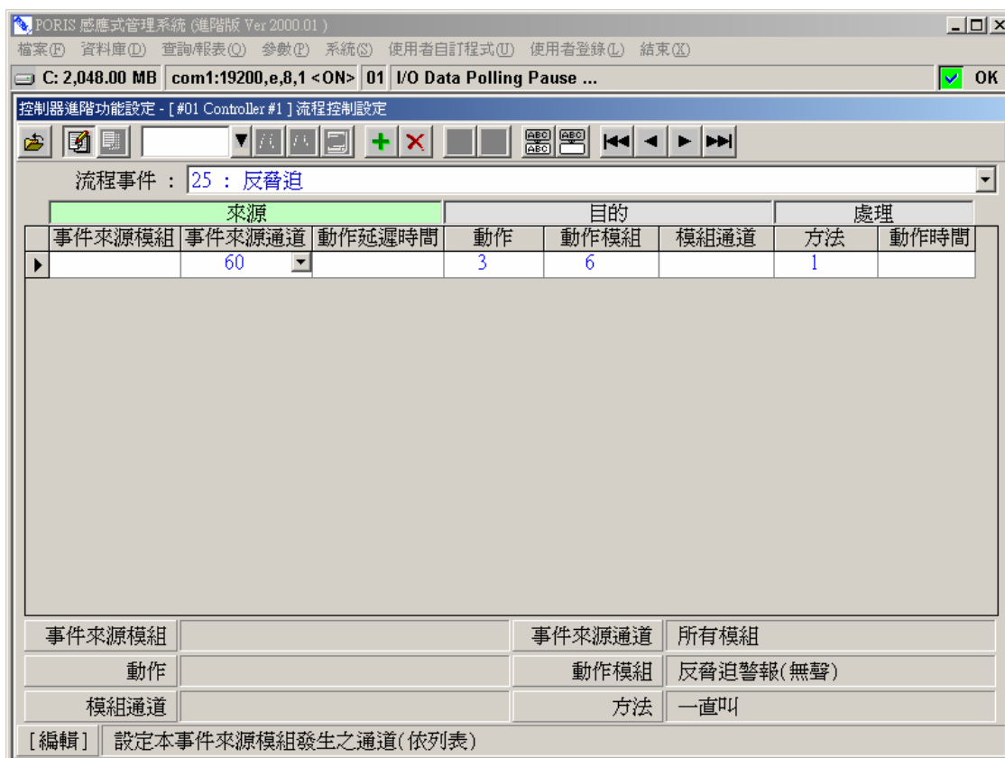
圖 2-25 流程事件 – 反脅迫
