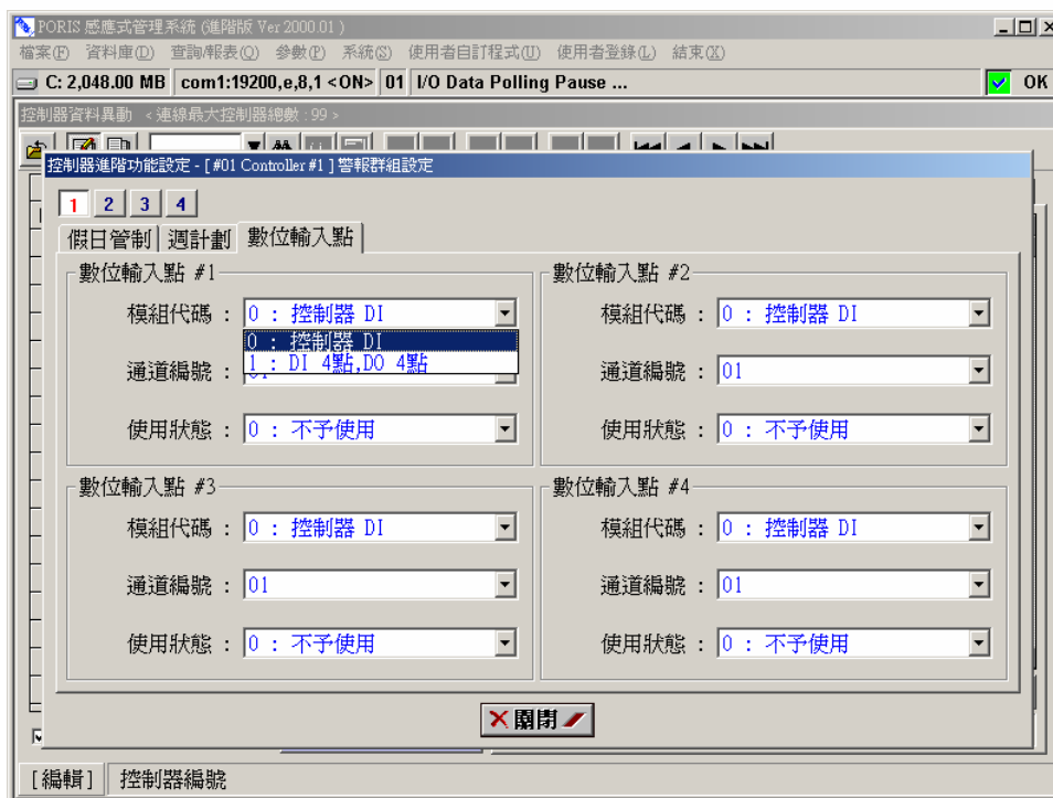
圖 4-6 警報群組 – 模組代碼選擇
