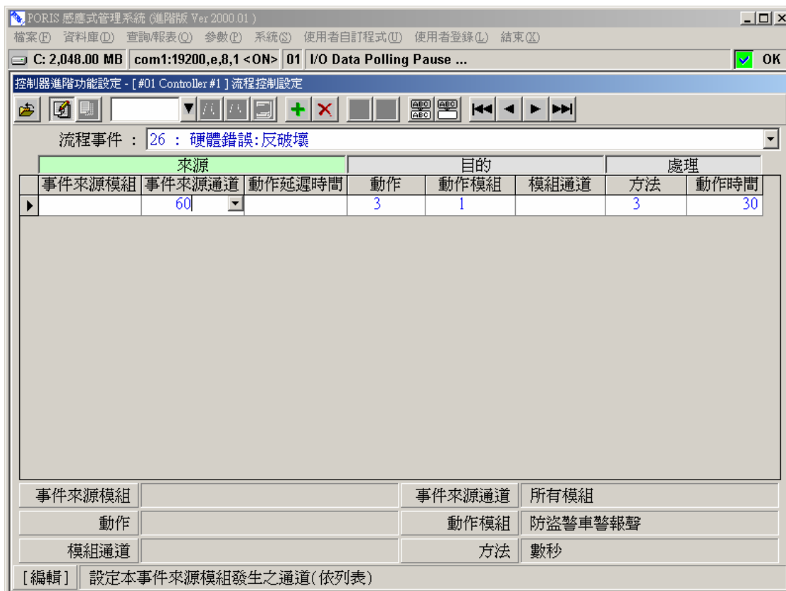
圖 2-26 流程事件 – 硬體破壞-反破壞
