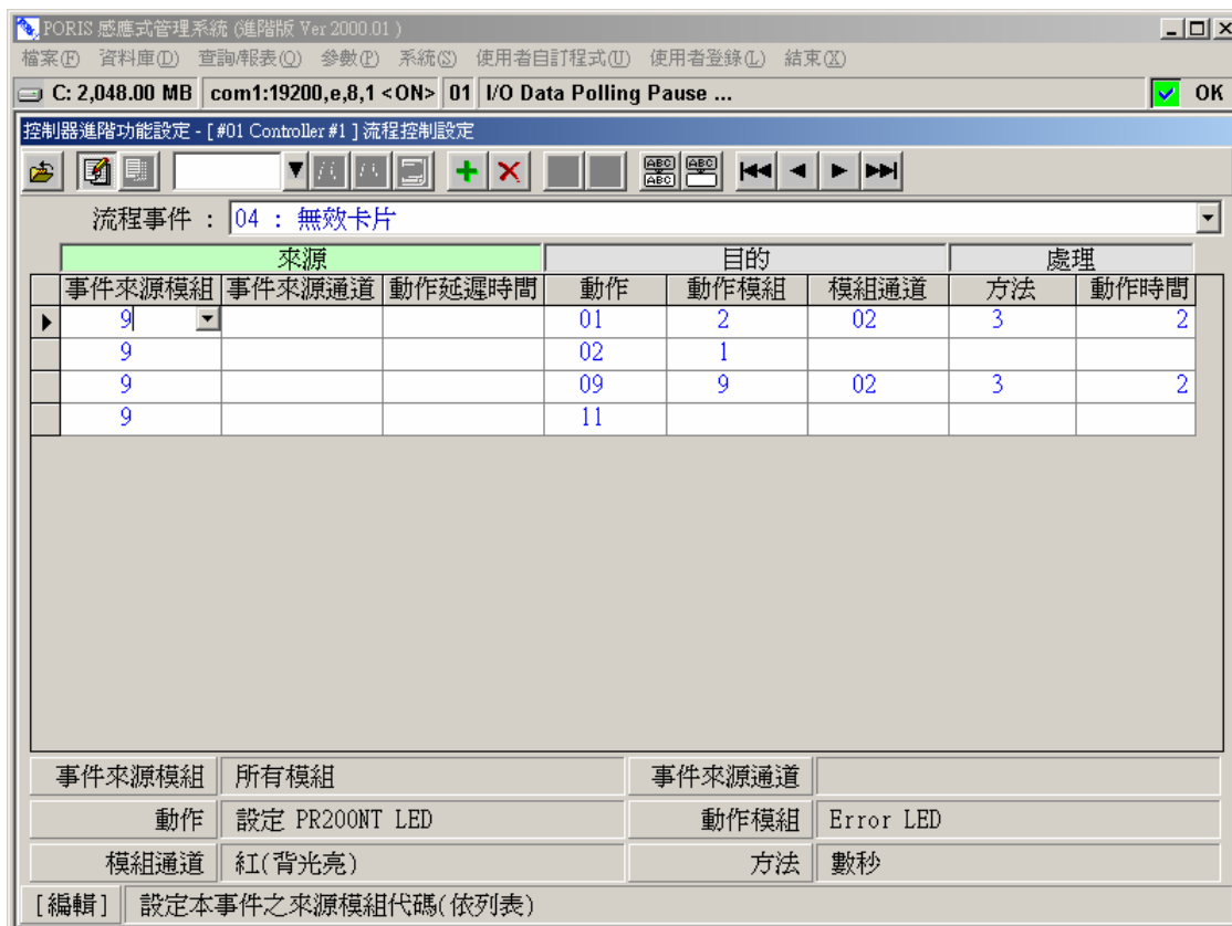
圖 2-4 流程事件 – 無效卡片
