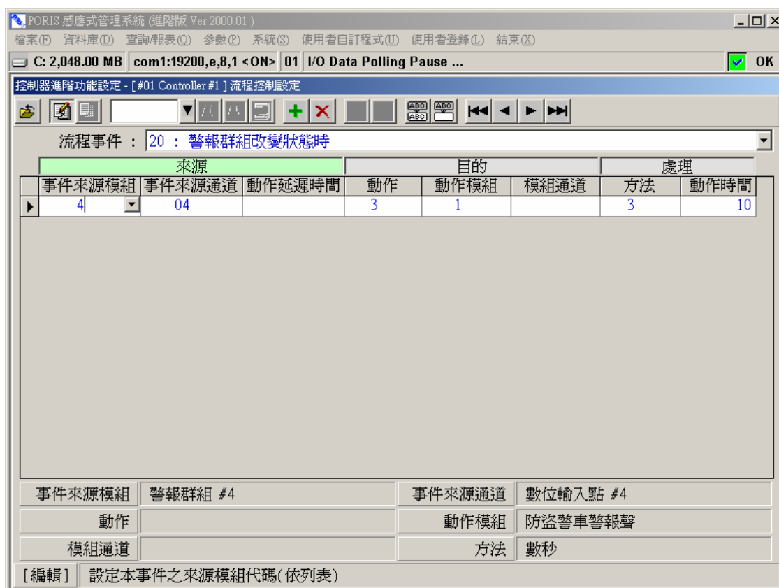
圖 2-20 流程事件 – 警報群組狀態改變時
