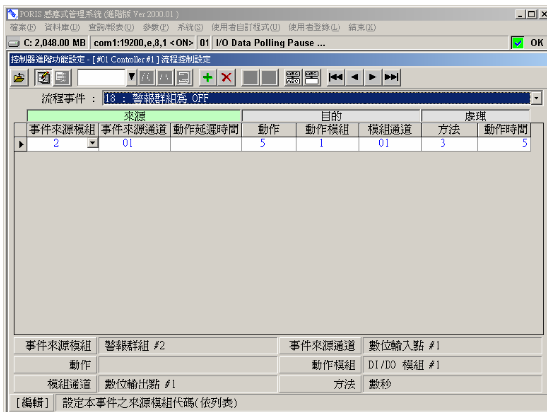
圖 2-18 流程事件 – 警報群組為 OFF
