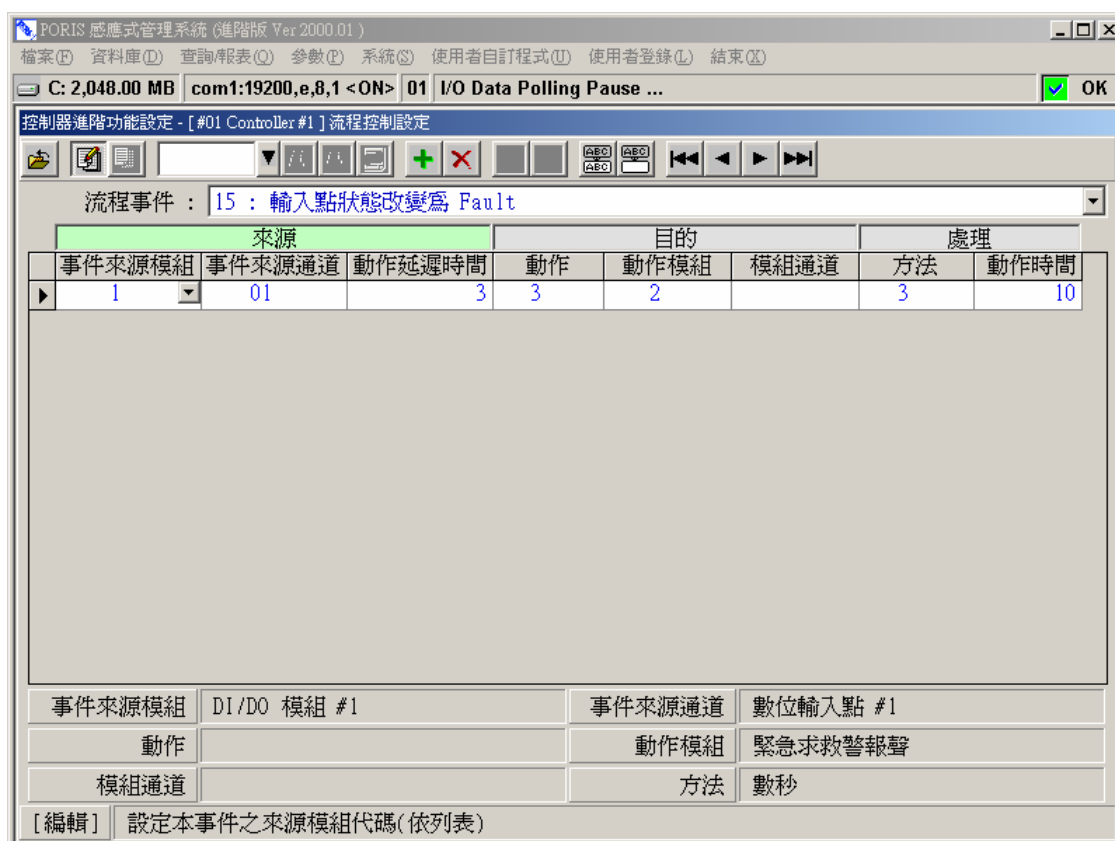
圖 2-15 流程事件 – 輸入點狀態改變為 Fault
