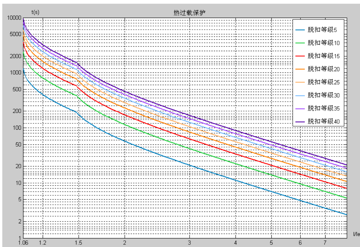
十五. 附表二：增安型电机 tE 时间保护特性表
