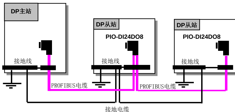
图3 设备接地示意图
