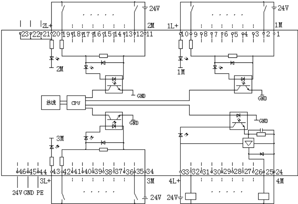
图 7 PIO-DI24DO8 接线图
