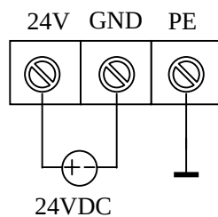
图2 PIO-DI24DO8 一体机电源端子图
