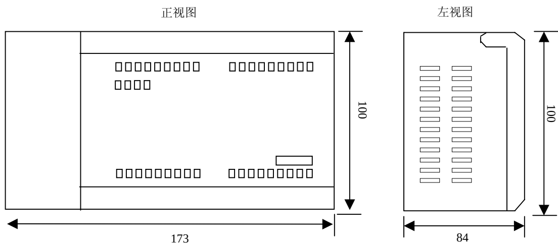
图6 PIO-DI24DO8 产品的外形尺寸图
