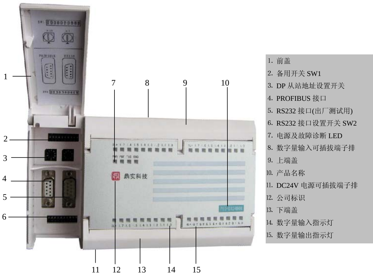
图 1 PIO-DI24DO8 产品外观图
