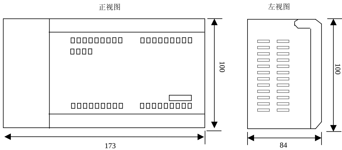
图 6 PIO-DI20DO12R2 产品的外形尺寸图
