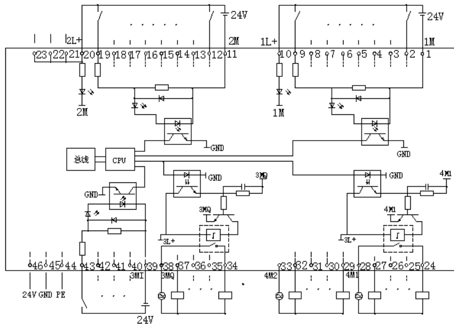
图7 PIO-DI20DO12R2 接线图
