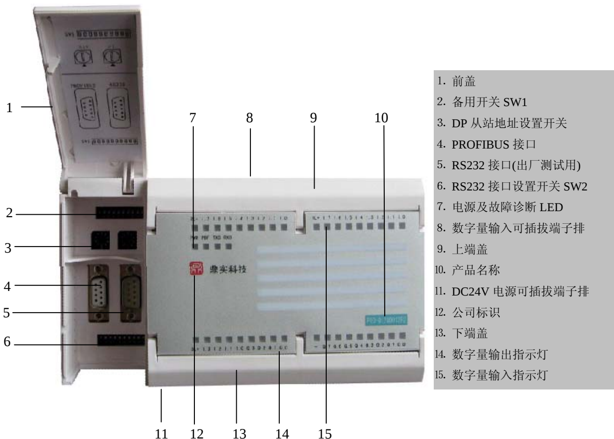
图 1 PIO-DI20DO12R2 产品外观图
