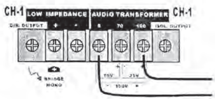
100 volt conexión de salida de línea
