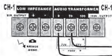
50 volt高电平输出连接
