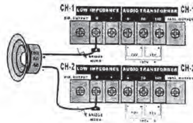
ICON300/700输出连接， 桥接Mono模式
