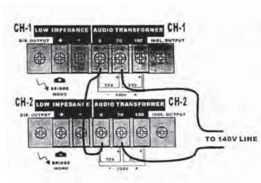
140 volt高电平输出连接，桥接单声道模式
