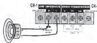
ICON300/700输出连接， 直流低阻抗
