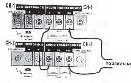
200 volt高电平输出连接，桥接单声道模式
