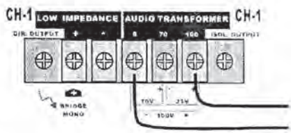
100 volt高电平输出连接
