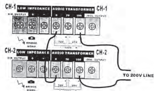
200 volt conexión de línea de salida, modalidad bridge mono.
