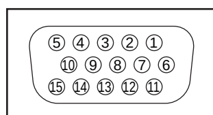
接头的信号名称
