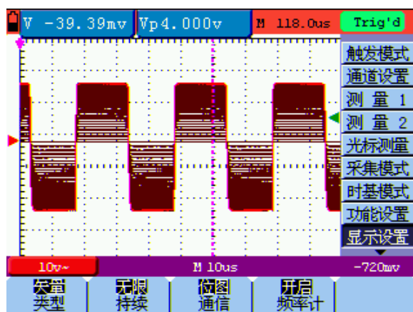
图 13：无限余辉显示
