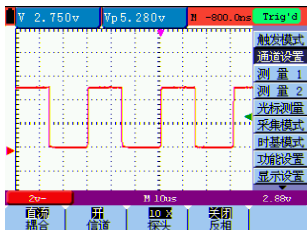
图 33: 直流耦合
