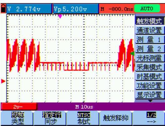
图37 视频指定行触发（第一页）
