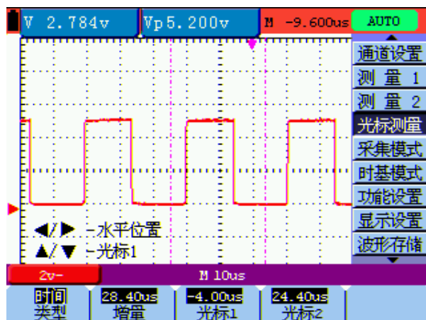
图 46: 光标时间测量
