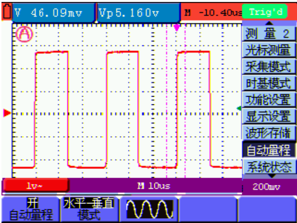
图 47 自动量程 水平---垂直模式多周期波形图
