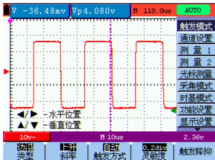
图 5：示波器菜单显示界面
