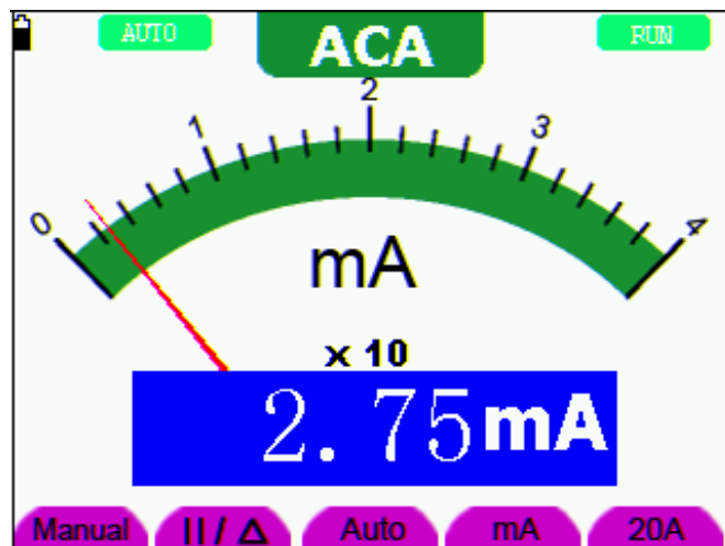
图 26: 交流电流测量界面
