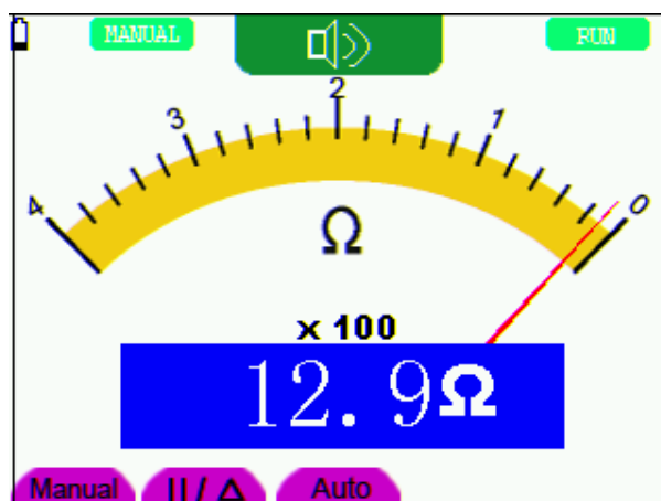
图 20：通断测量
