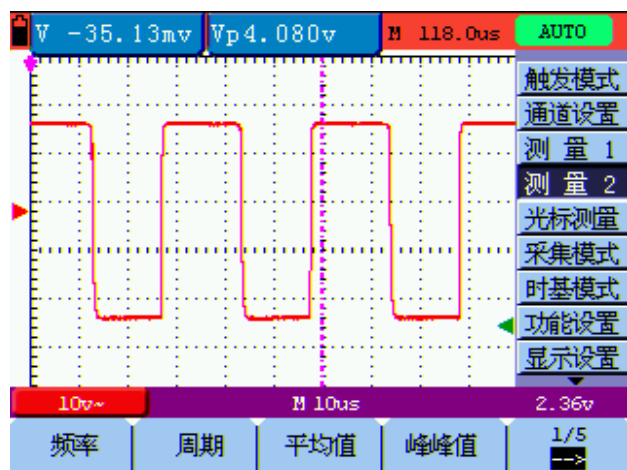
图 10：自动测量
