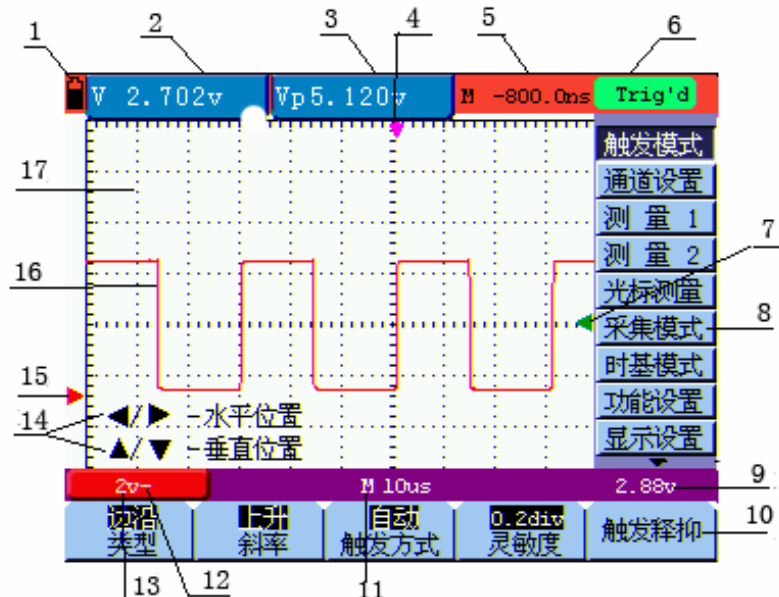
图 4: 示波器界面
