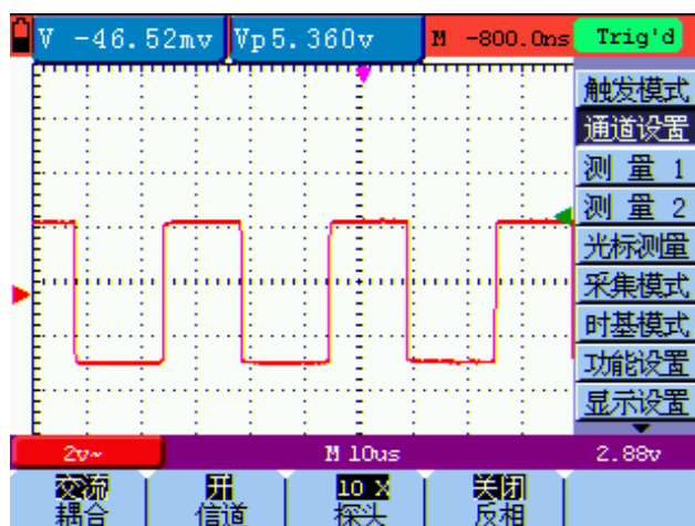
图 15: 交流耦合
