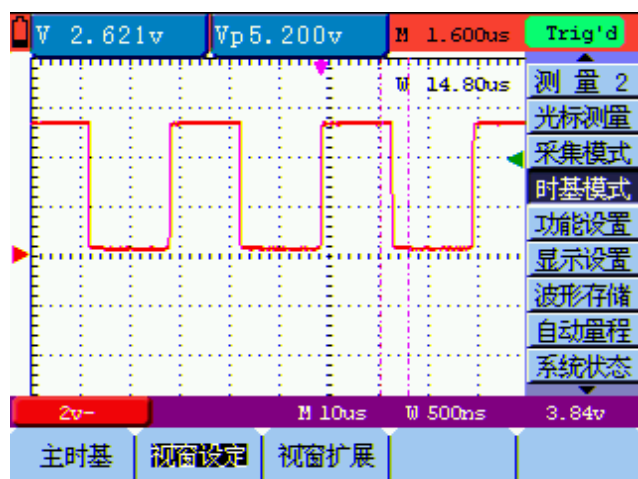
图49：视窗设定
