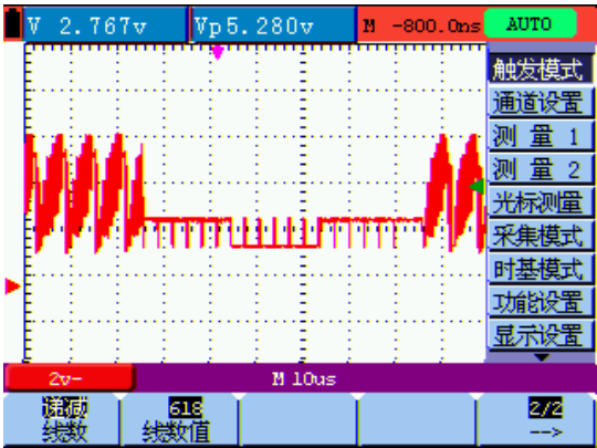
图38 视频指定行触发（第二页）
