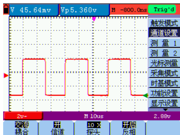
图 16: 反相开启
