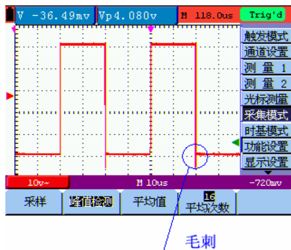
图 14：峰值检测
