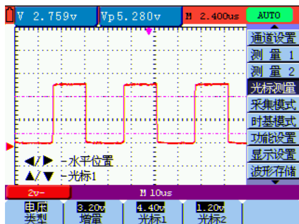
图 45: 光标电压测量
