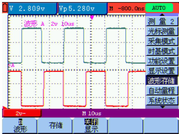
图 43：波形储存
