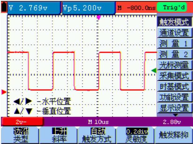
图 35：边沿触发
