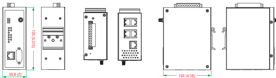
前/后视图
