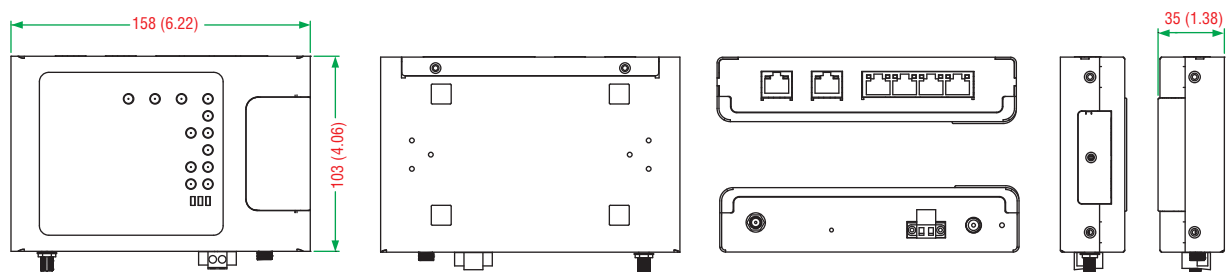
前/后视图
