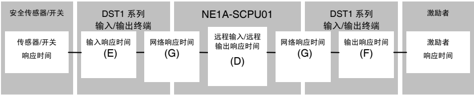
(4) 远程输入—远程输出
