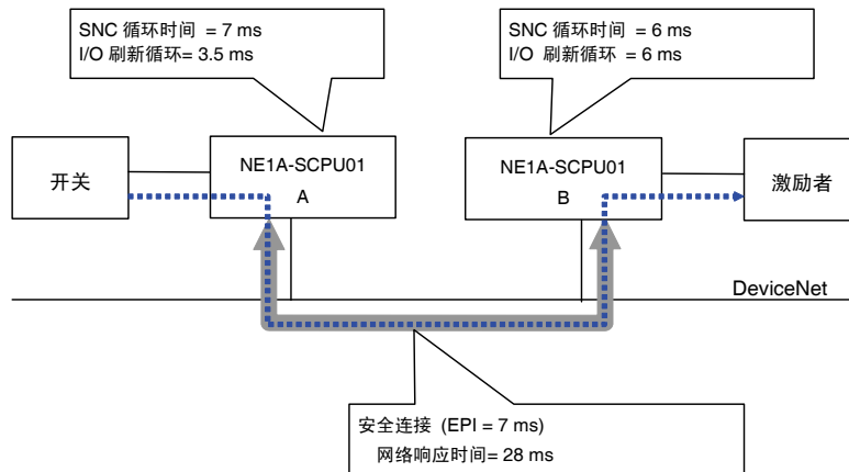
例 2: 本地输入—远程输出
