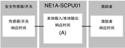
(2) 远程输入—NE1A-SCPU01 输出
