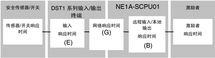
(3) NE1A-SCPU01 输入—远程输出
