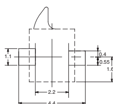
印刷基板焊盘尺寸图 (参考) (TOP VIEW)
