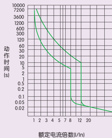
图9 NM7-630动作特性曲线
