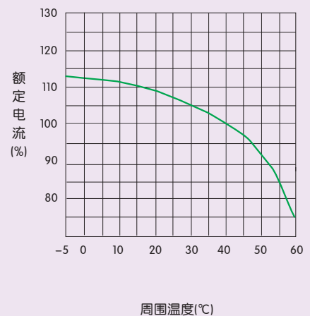
图12 NM7-800温度补偿曲线
