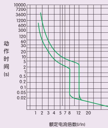
图9 NM7-630动作特性曲线
