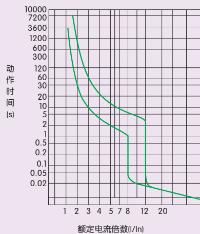
图1 NM7-63(10A~32A)/NM7-125(16A~32A)动作特性曲线
