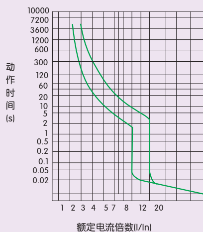
图11 NM7-800动作特性曲线
