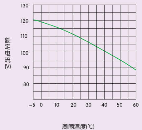
图10 NM7-630温度补偿曲线
