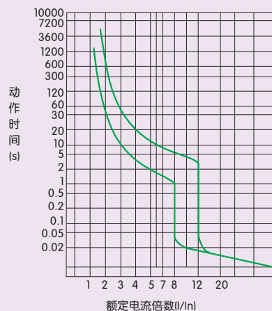
图3 NM7-63(40A~63A)/NM7-125(40A~125A)动作特性曲线
