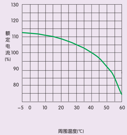
图10 NM7-630温度补偿曲线
