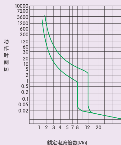
图5 NM7-250动作特性曲线
