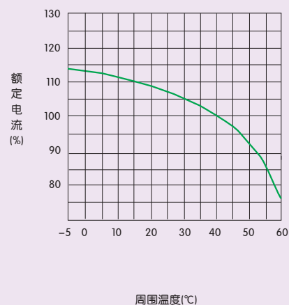
图6 NM7-250温度补偿曲线
