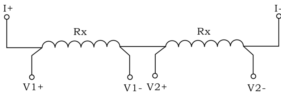
双通道测量
