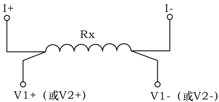
单通道测量
