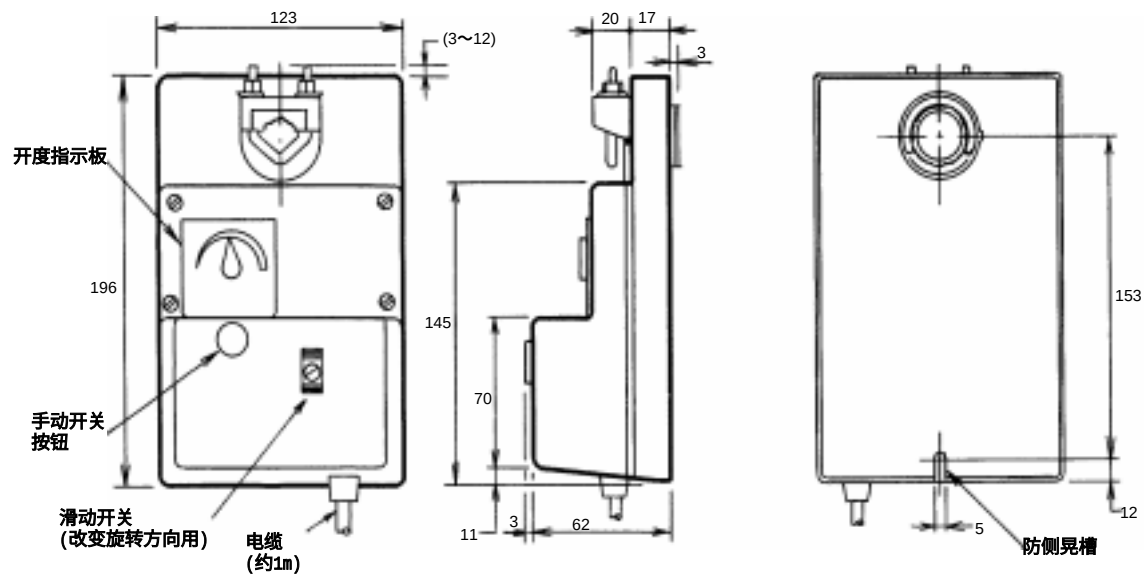
图1 外形尺寸(mm)
