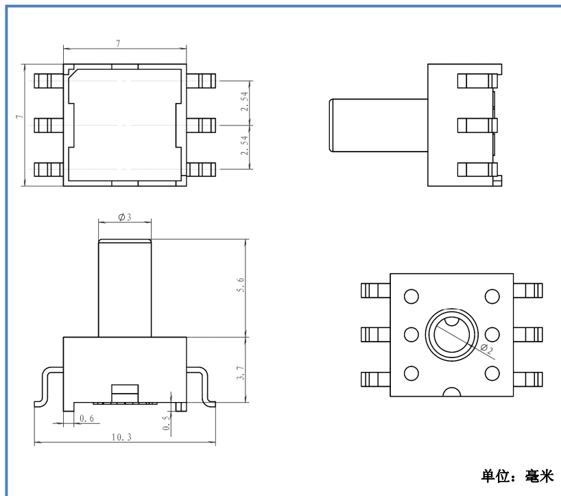
图四 GSR 型封装机械尺寸与外观图
