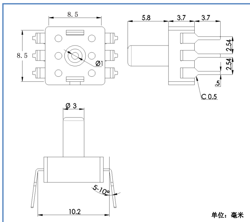
图五 GDR 型封装机械尺寸与外观图
