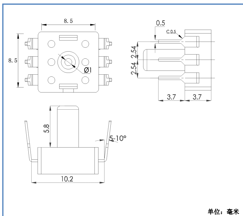
图六 GDF 型封装机械尺寸与外观图
