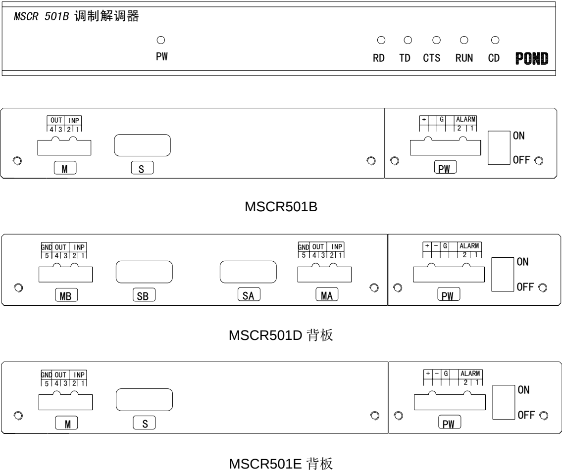
图 1 MSCR501 前、背面板布置图
