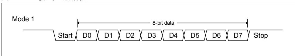
图 133-1 模式 1 数据帧
