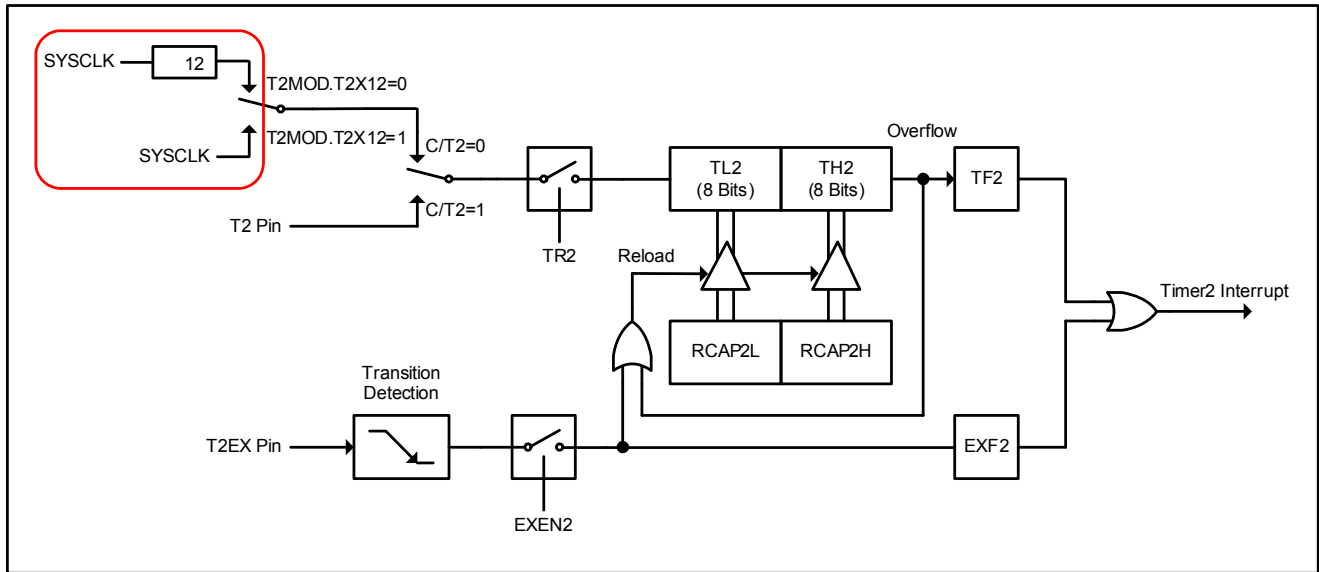
图 12-6 定时器 2 自动加载模式 (CEN=0)
