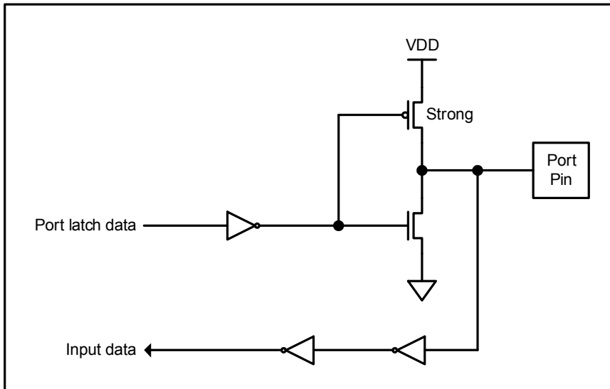
图 10-2 推挽输出
