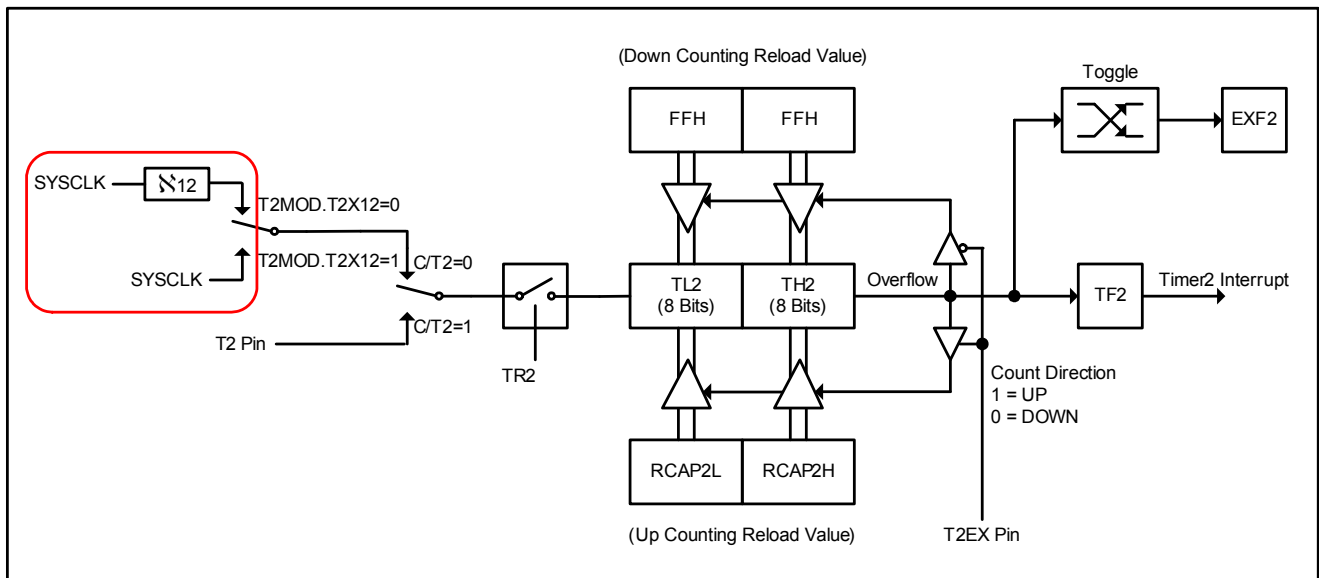
图 12-7 定时器 2 自动加载模式 (CEN=1)
