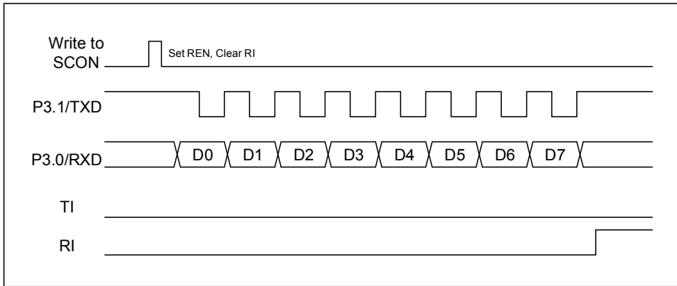
图 133-5 模式 0 接收波形
