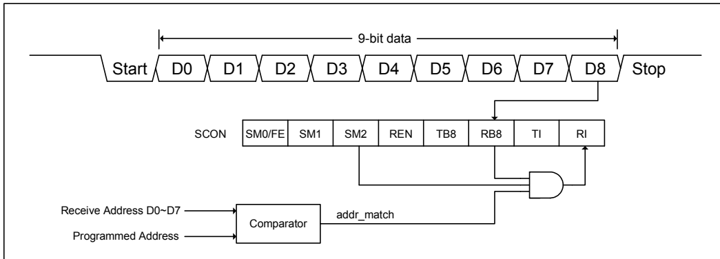
图 133-9 自动地址识别
