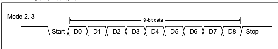
图 133-2 模式 2 数据帧
