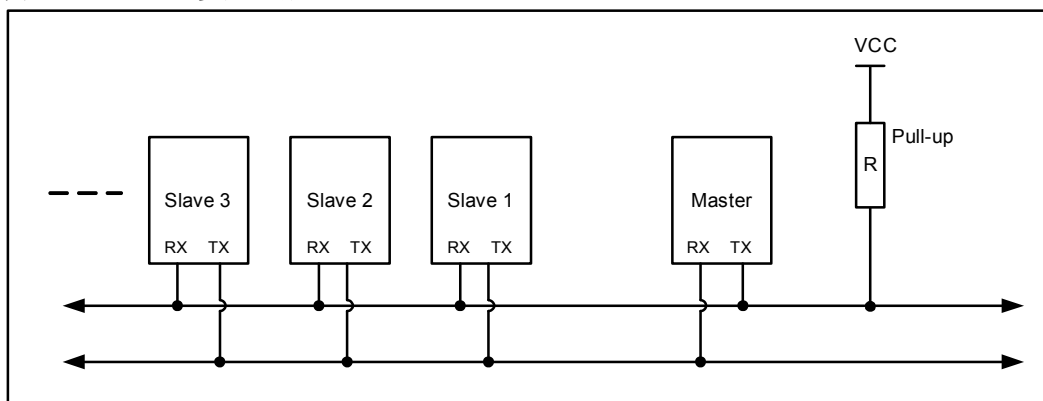
图 133-8 UART 多处理器通讯
