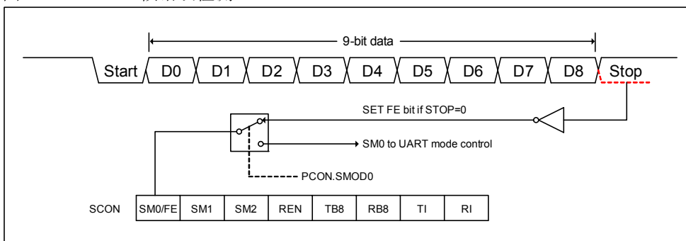
图 133-7 UART 帧错误检测
