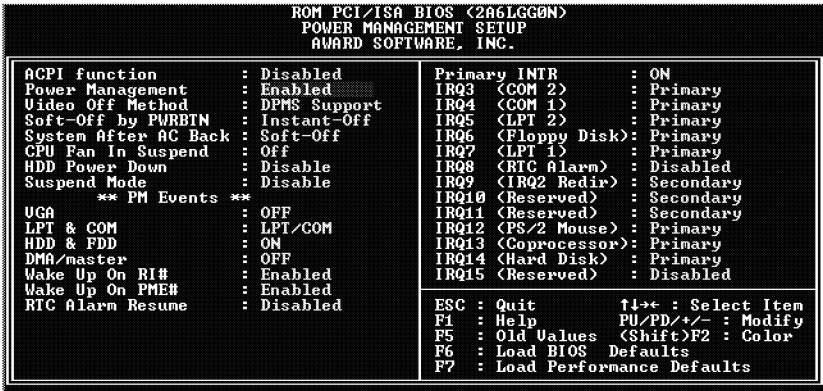
图 - 5 电源管理设置
