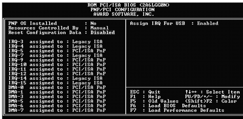
图 - 6 PNP/PCI 参数设置
