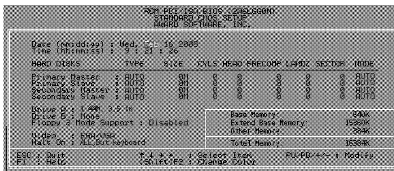
图 - 2 基本 CMOS 参数设置
