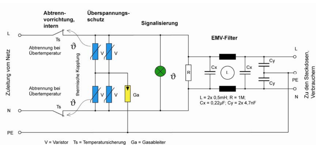
Fig. 1 Schaltbild Überspannungsschutz und EMV-Filter
