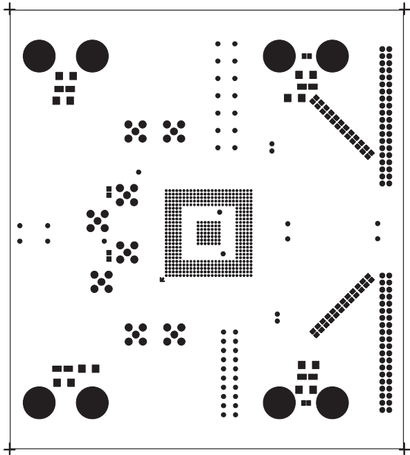
Figure 6e. Layer 3
