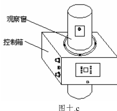
图十: 控制箱安装示意图
