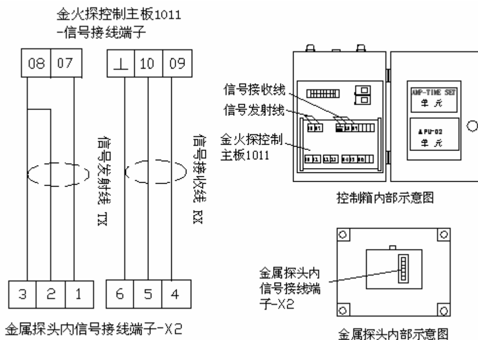
图八：金探信号连接图
