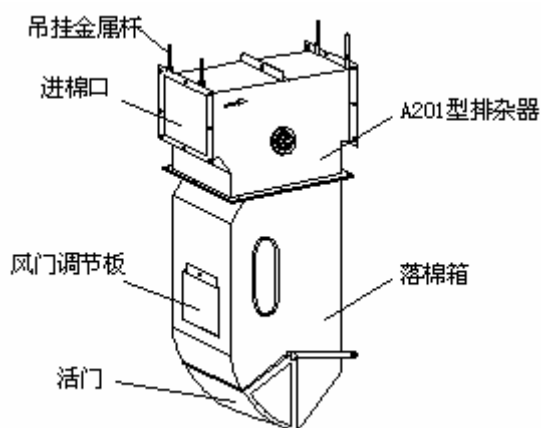
图十二：排杂执行机构安装示意图
