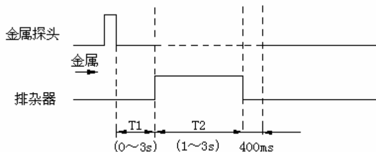
图十五.a 金探动作状态图
