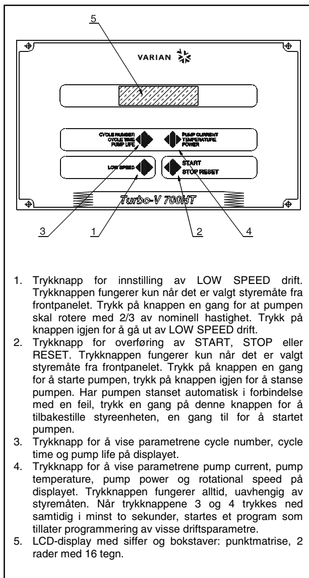
Frontpanelet på styreenheten 969-9445 og 969-9545
