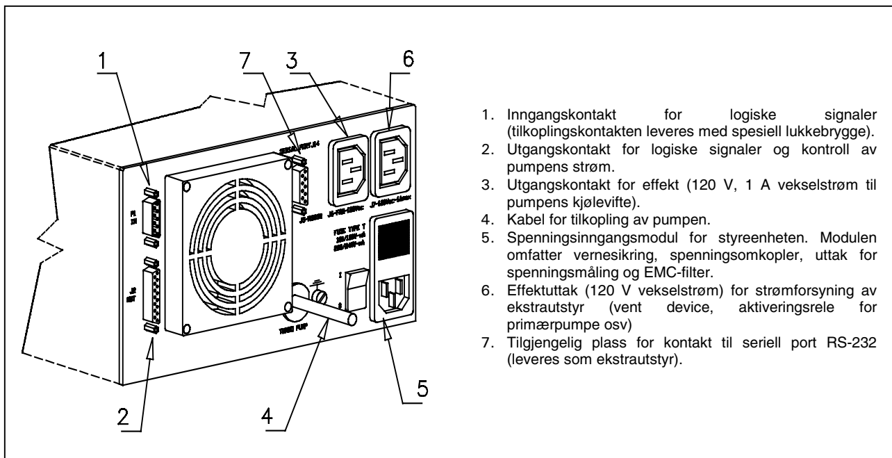
Bakpanelet på styreenheten 969-9445 og 969-9545
