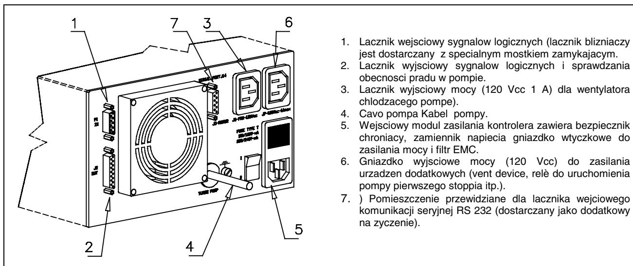
Pulpit tylny kontrolerów 969-9445 I 969-9545
