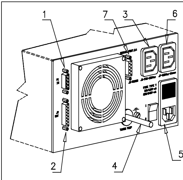
Panel trasero del controlador 969-9445 y 969-9545
