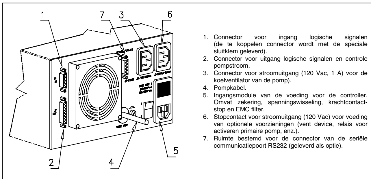
Achterpaneel van de controllers 969-9445 en 969-9545
