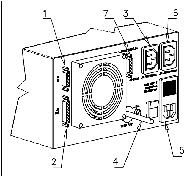
Rückseitige Tafel der Controller 969-9445 und 969-9545
