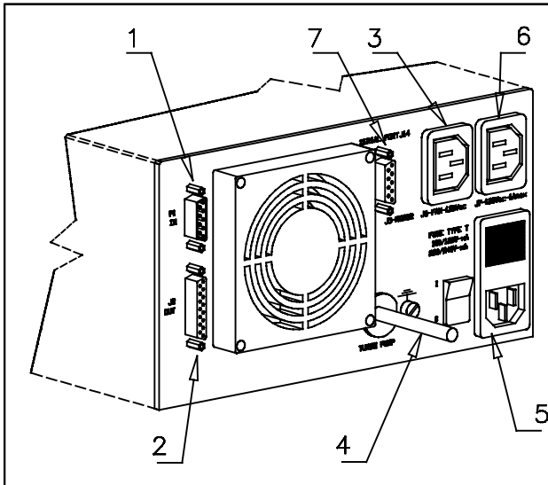
Ozadnja plošča controllerjev 969-9445 in 969-9545
