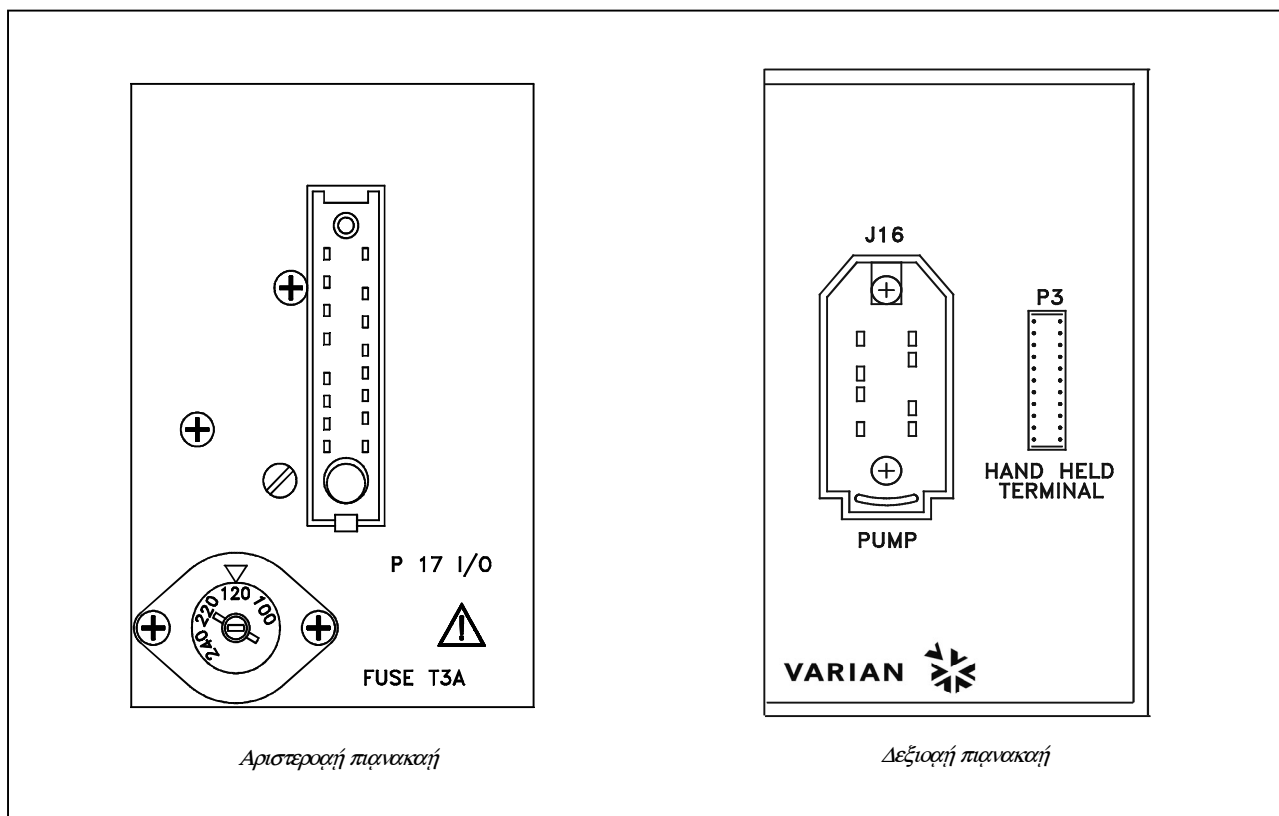
Δεξιοή και αριστεροή πινακακή του Ρυθμιστή 969-9504
