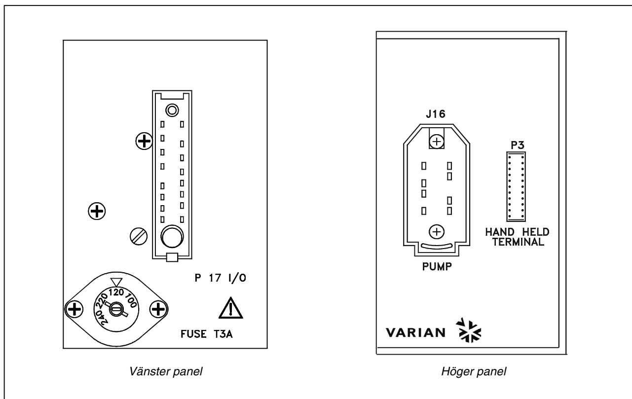
Vänster och höger panel på Styrenheten 969-9504
