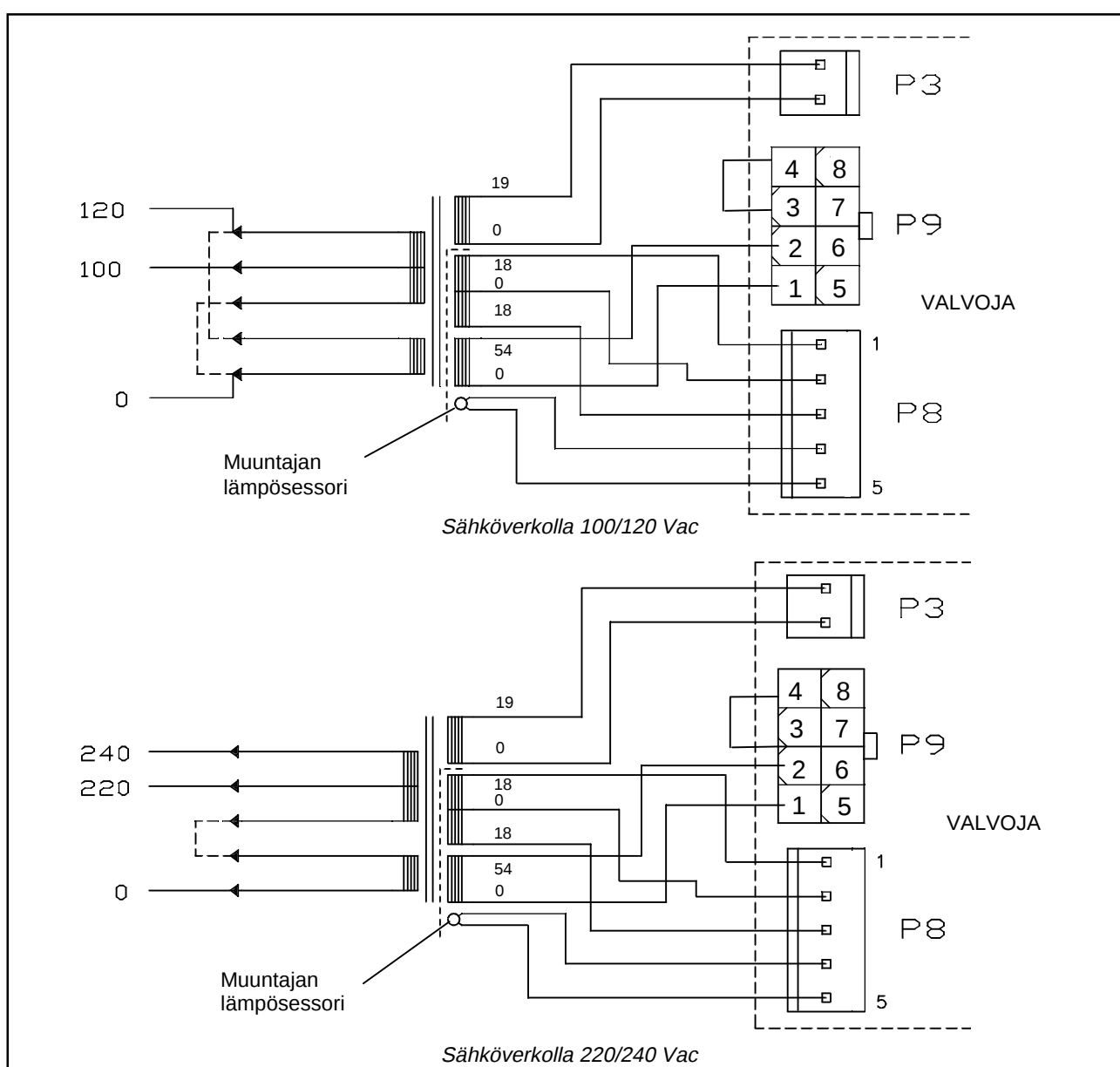
Kytännät valvojan, sähkömuuntajan ja sähköverkon välillä
