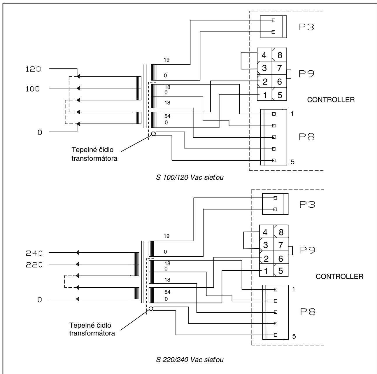
Prepojenia medzi Controllerom, Napájacím Transformátorom a Siet'ou
