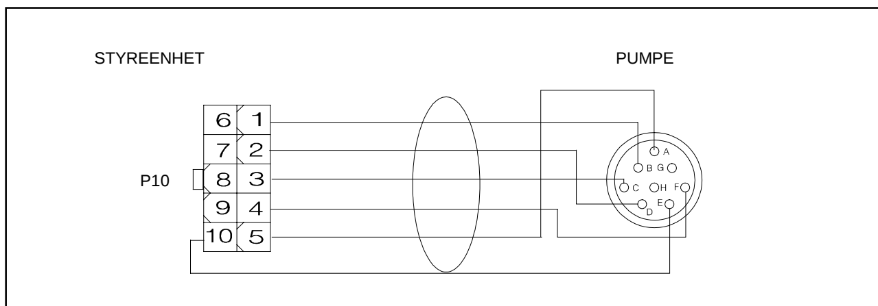
Forbindelseskabel mellom styreenheten og pumpen
