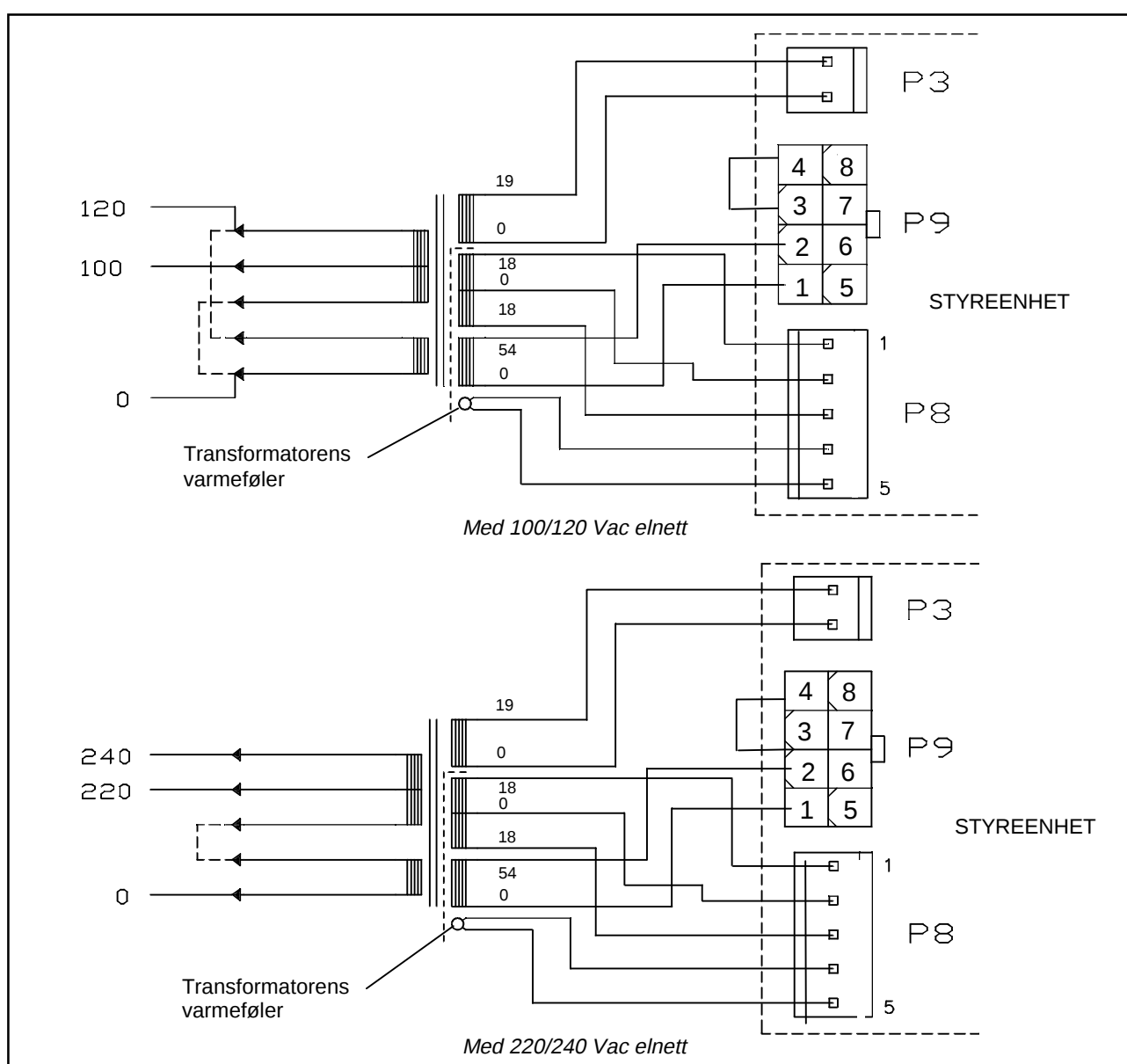
Forbindelser mellom styreenheten, effektransformatoren og elnettet
