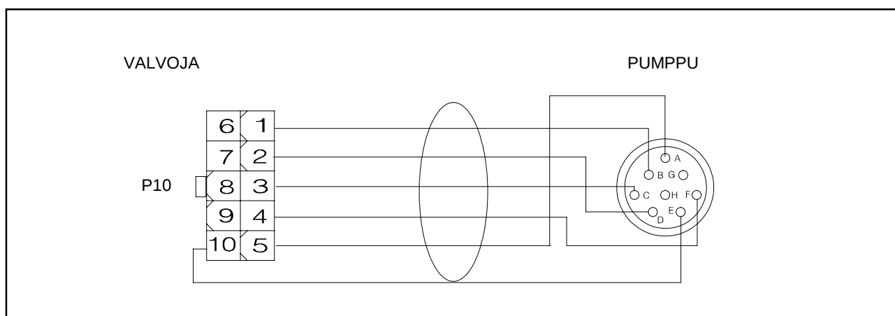
Liitoskappeli valvojan ja pumpun välillä
