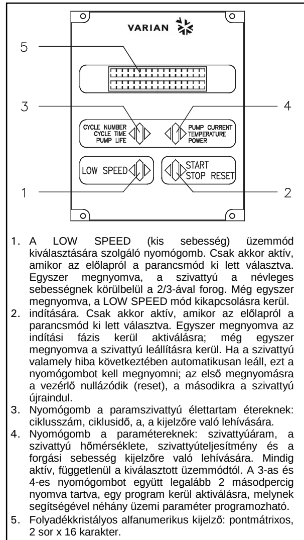
A Hand Held Terminal előlapja
