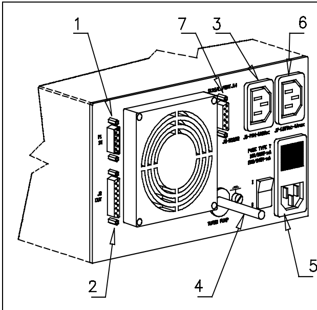
Rückseitige Tafel der Controller 969-9454 und 969-9554
