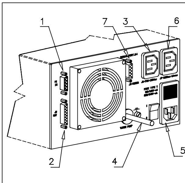
Pulpit tylny kontrolerów 969-9454 i 969-9554
