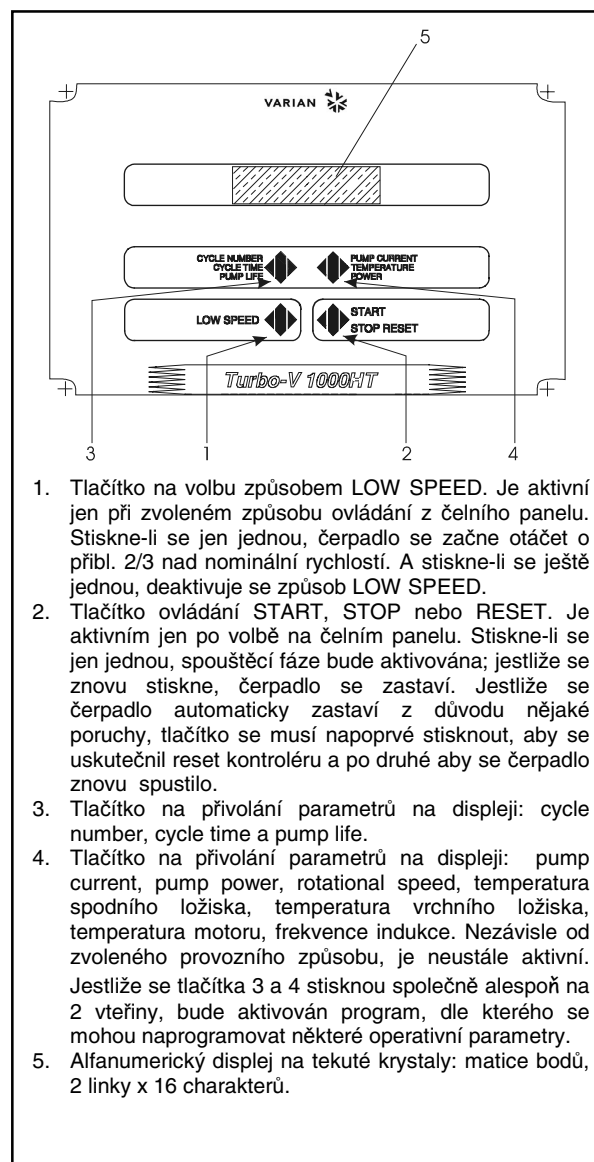
Čelní panel Kontroléru 969-9454 a 969-9554
