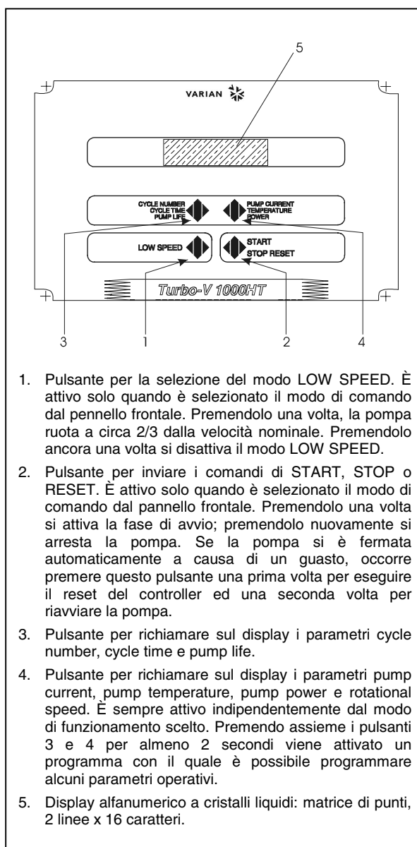
Pannello frontale del Controller 969-9454 e 969-9554
