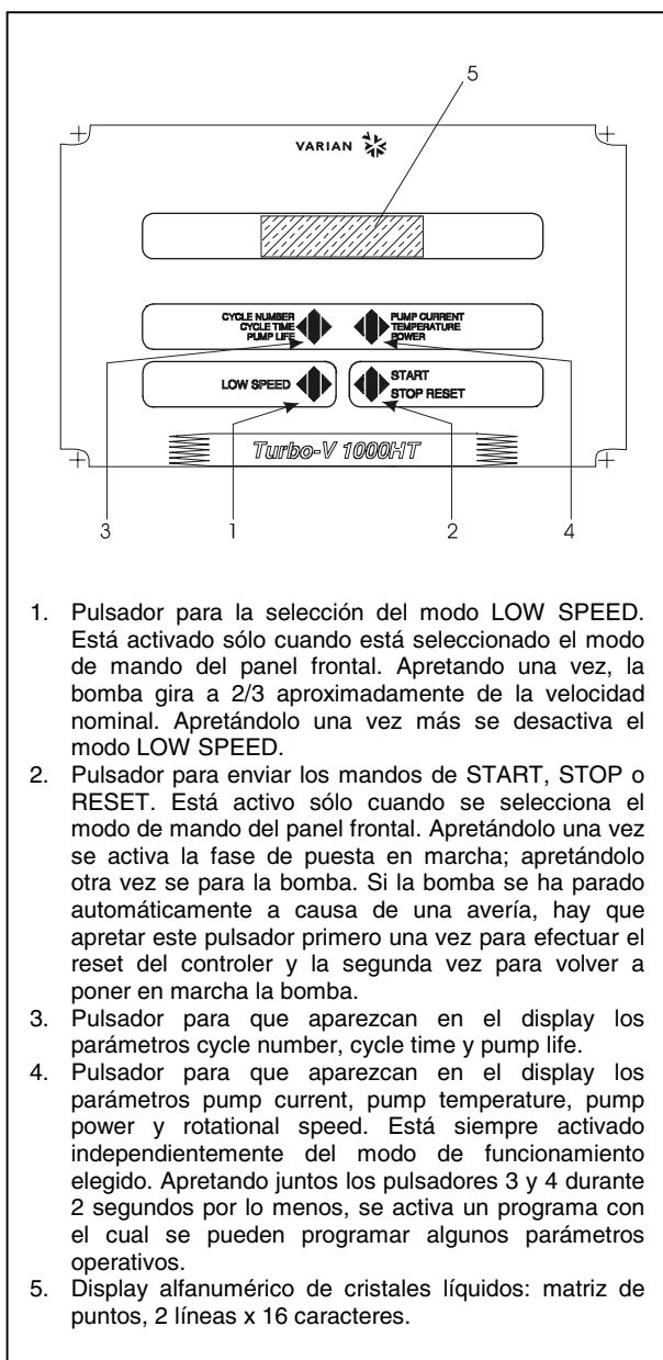
Panel frontal del controler 969-9454 y 969-9554
