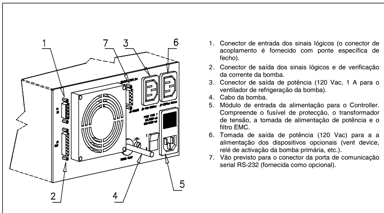
Painel posterior dos Controllers 969-9454 e 969-9554
