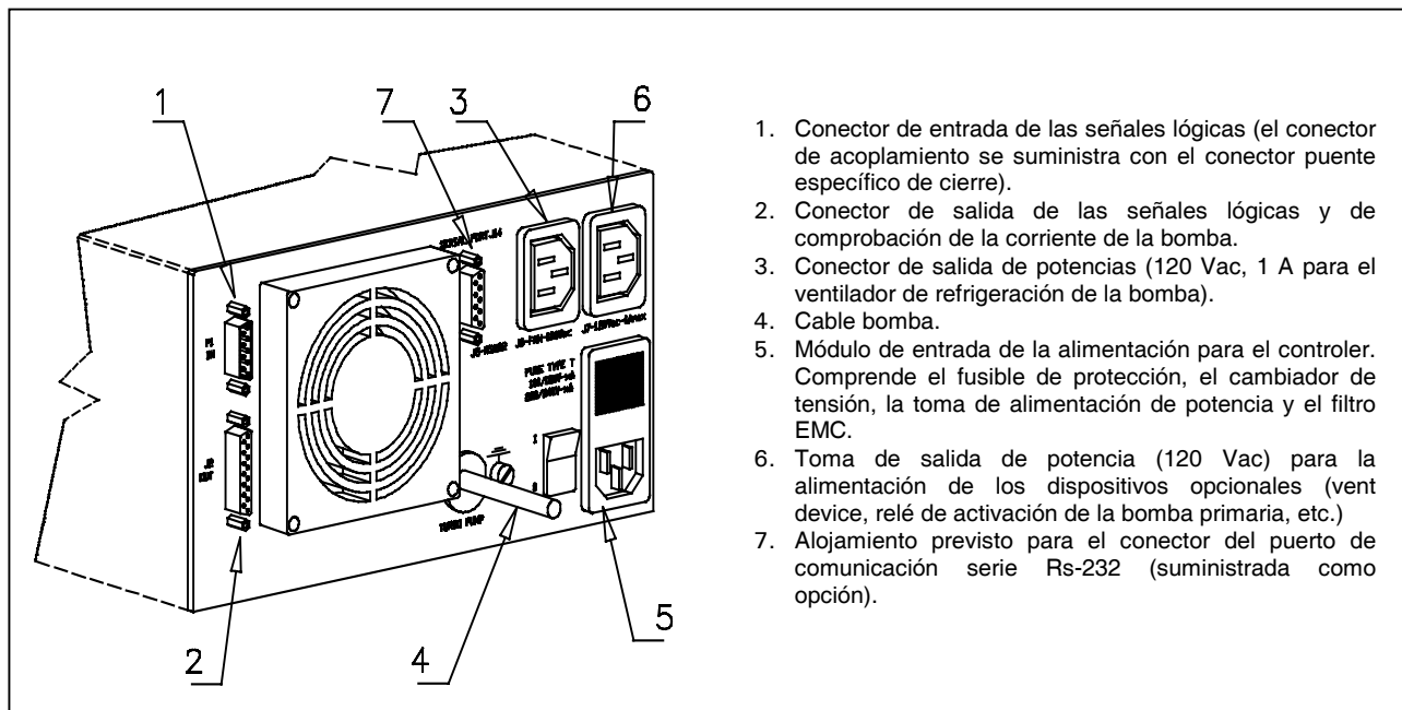
Panel trasero del controlador 969-9454 y 969-9554
