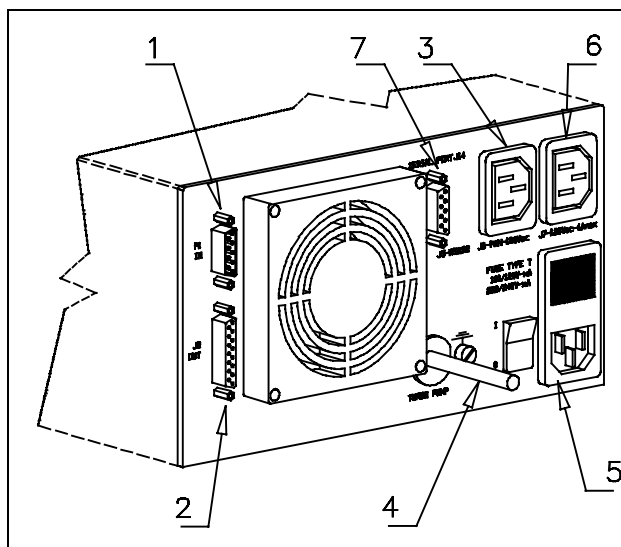
Pannello posteriore dei controller 969-9454 e 969-9554
