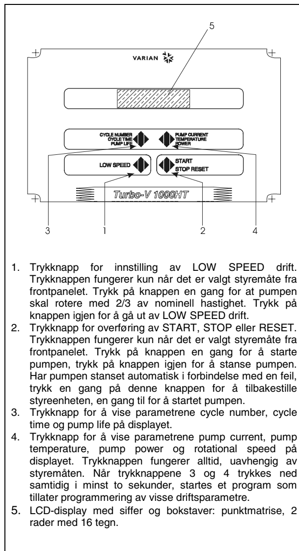
Frontpanelet på styreenheten 969-9454 og 969-9554
