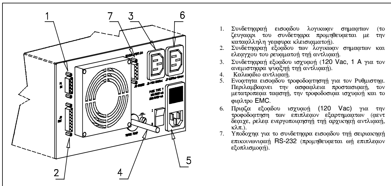
Εμπροσθιοή πινακιά του Ρυθμιστή 969-9454 και 969-9554
