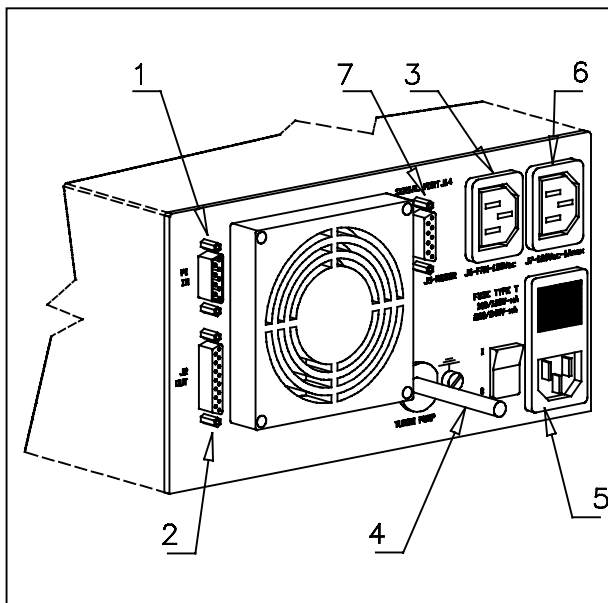
Ozadnja plošča controllerjev 969-9454 in 969-9554
