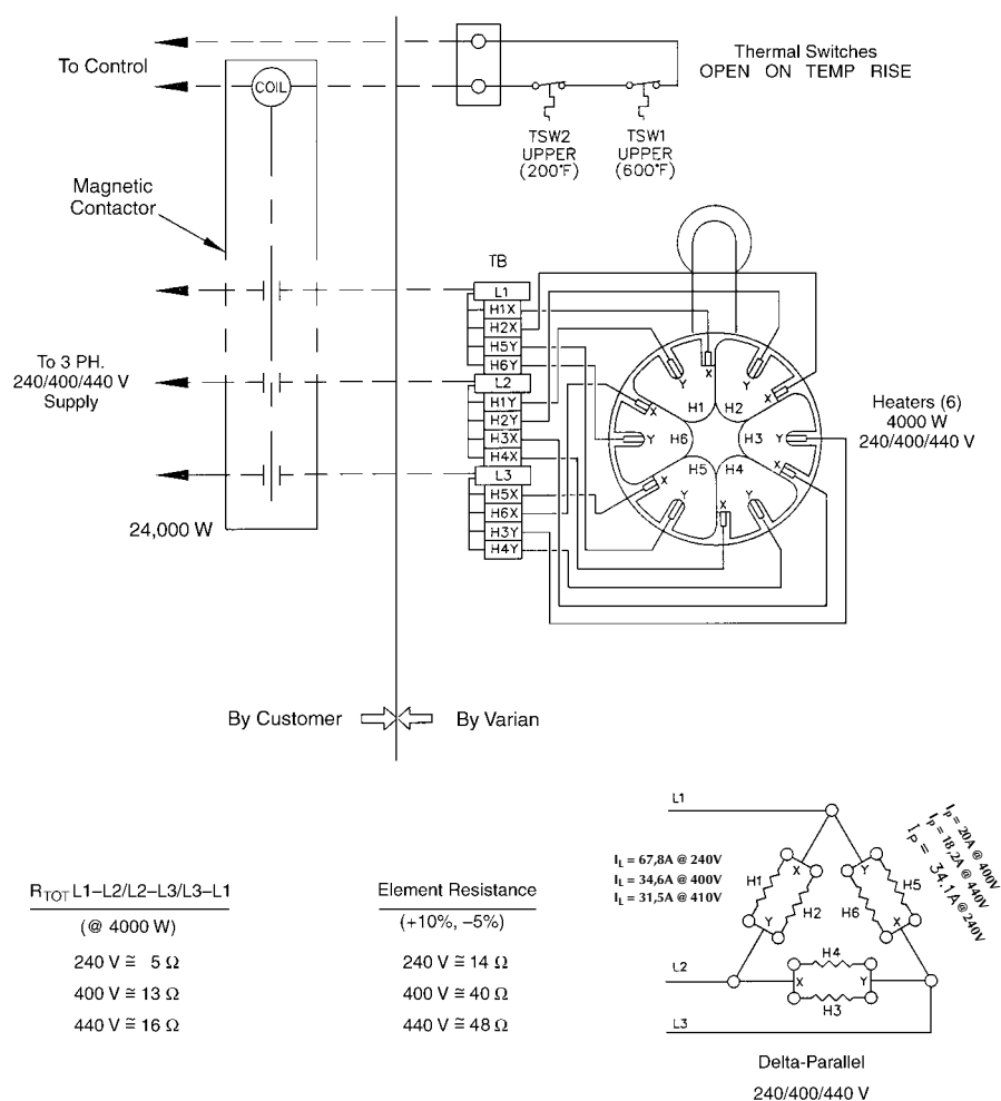
Figura 20 Schema elettrico delle pompe HHS-35 da 240/400/440 V
