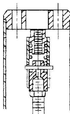
Dettaglio A Posizione degli accoppiamenti de prima del montaggio della copert
