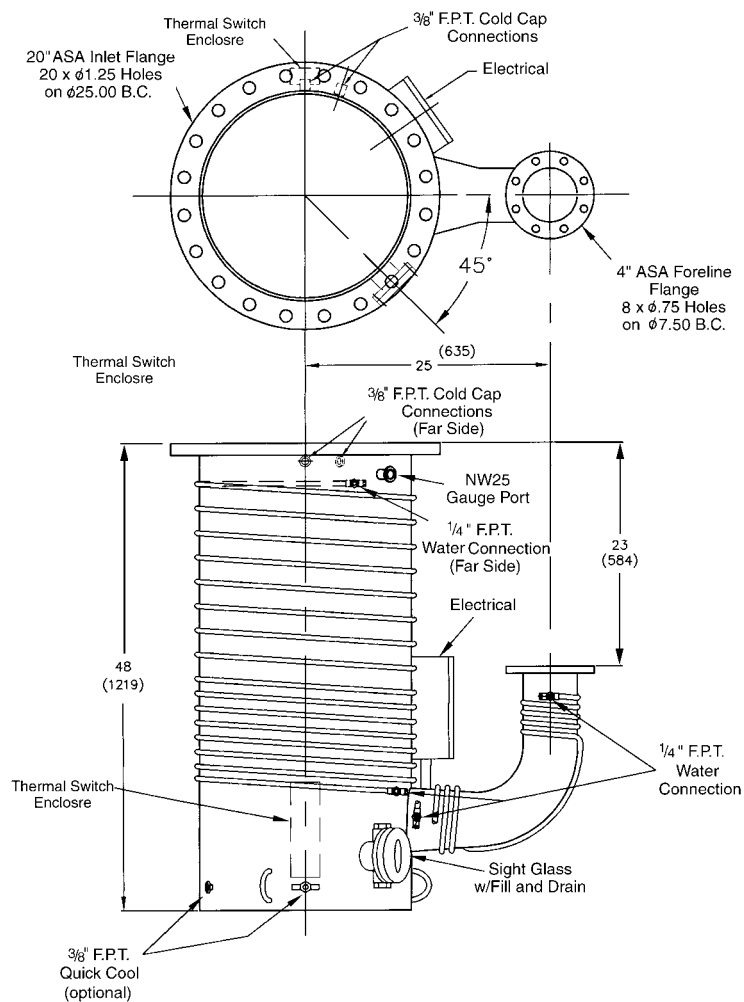
Figura 7 Vista della pompa HS-20 con flange ASA
