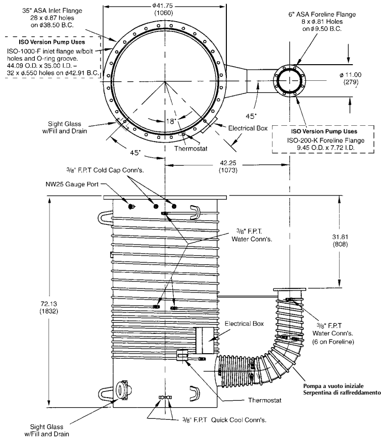
Figura 9 Vista della pompa NHS-35 con flange ASA
