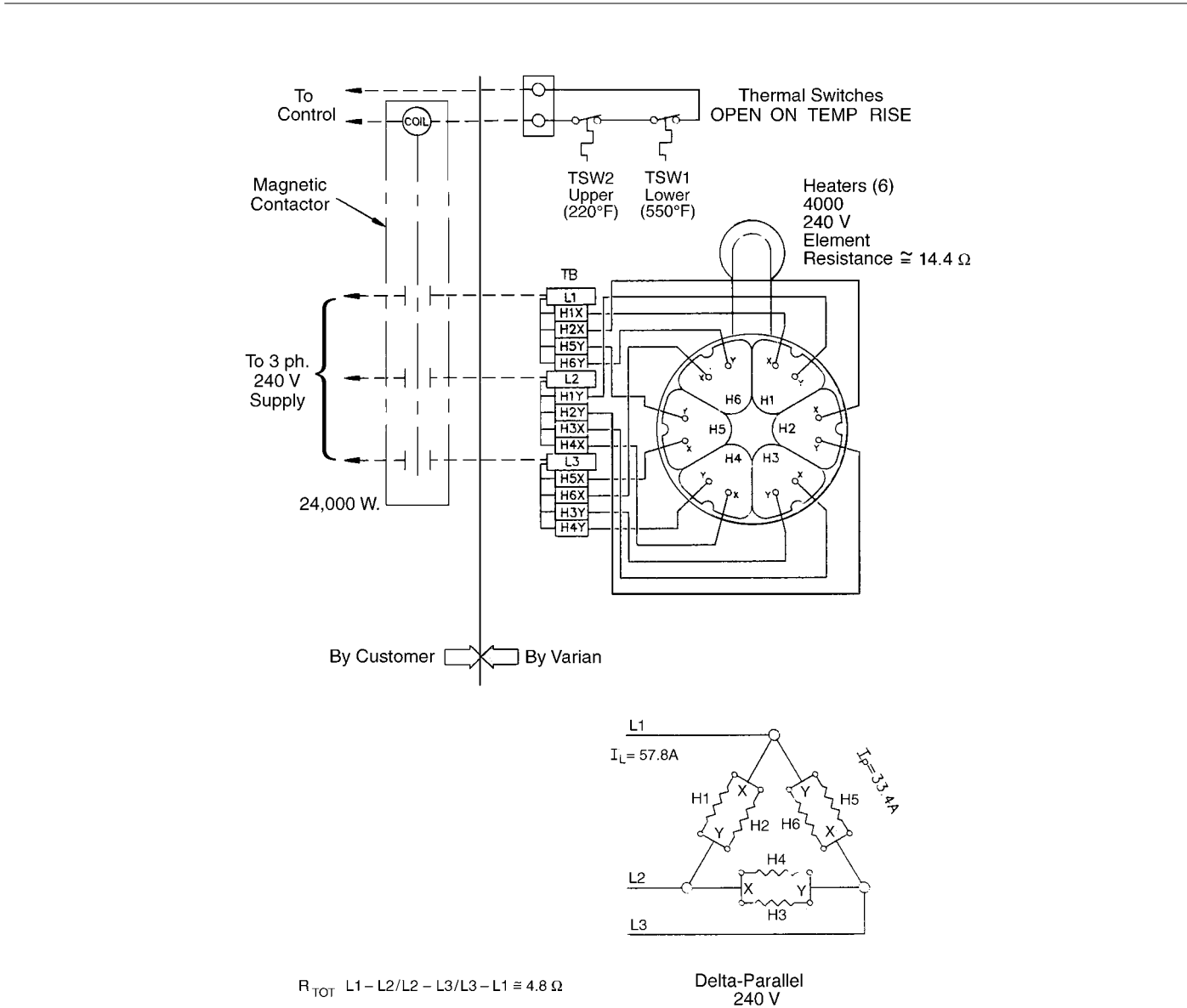
Figura 16 Schema elettrico delle pompe HS-32 da 240 V
