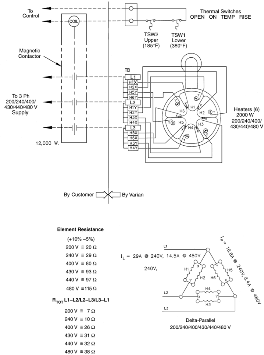
Figura 13 Schema elettrico delle pompe HS-20 da 200/240/400/430/480 V
