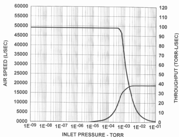
Figura 5 Curve della velocità e della capacità del modello HS-35
