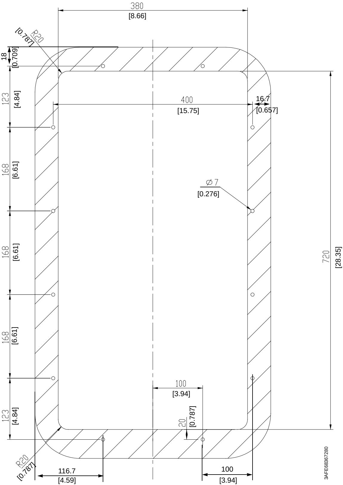
用于外形尺寸 R6 的法兰安装套件
