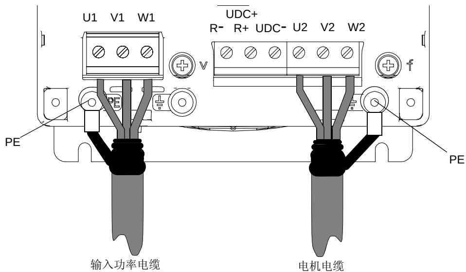
外形尺寸 R2 到 R4
