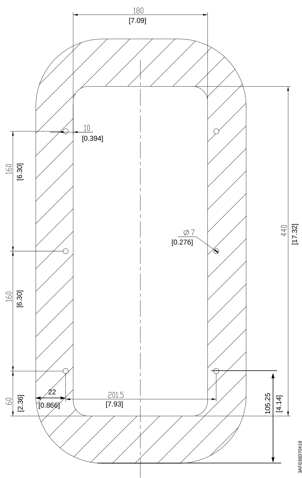
用于外形尺寸 R3 的法兰安装套件
