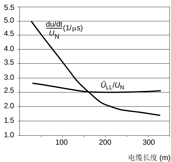
无 du/dt 滤波器
