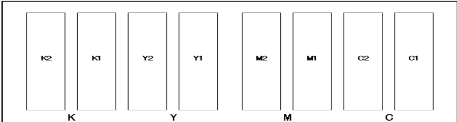
图 3-7 8 喷头排列图
