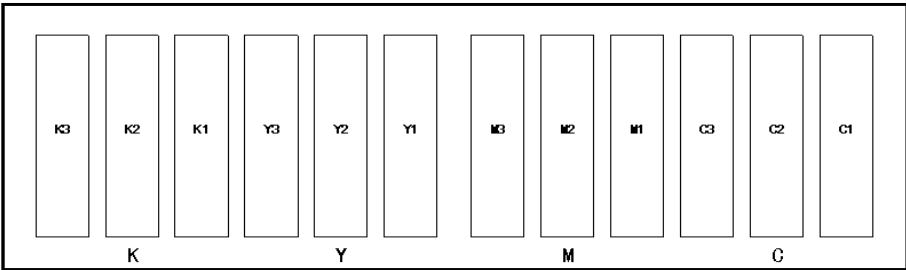
图 3-8 12 喷头排列图
