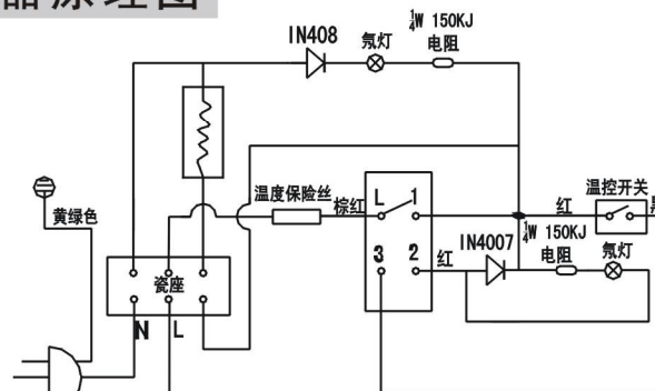
JYZS-M201电器原理图
