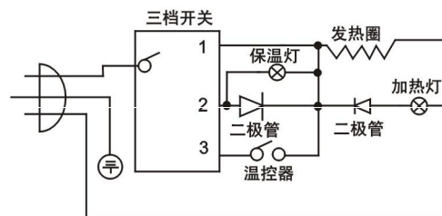
JYZS-M2501/M3501/M501电器原理图
