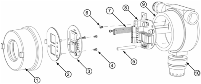
图8. 装配图
