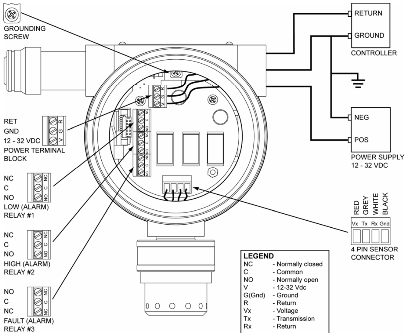
图5. 系统布线图
