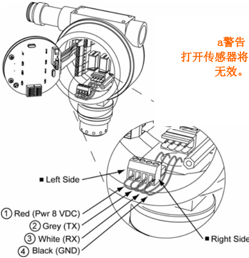
图9. 传感器布线图
