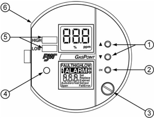
图2. 用户界面
