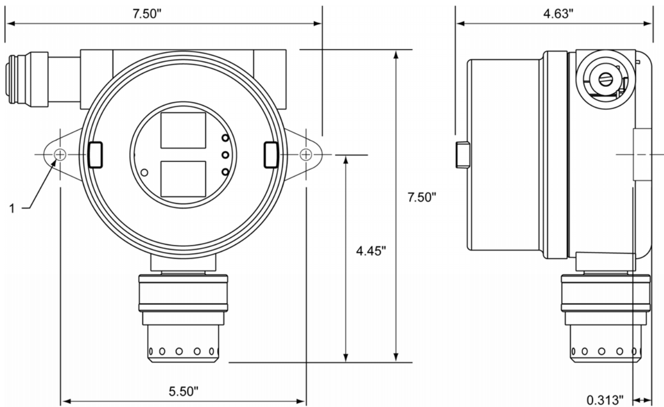
图4. 外形图
