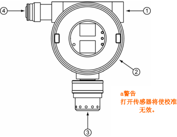
图1. GasPoint监控器
