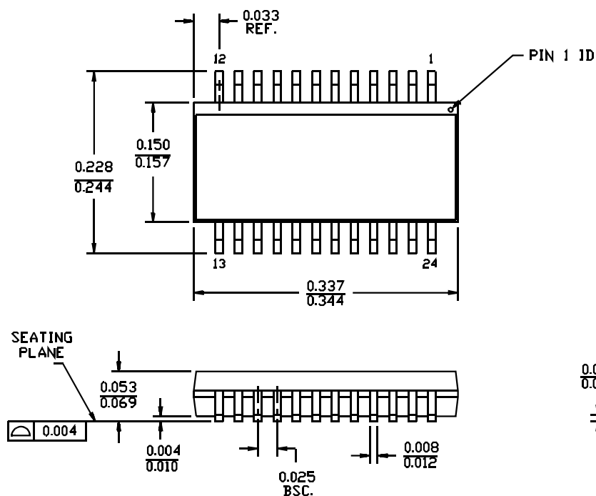
24-Lead Quarter Size Outline Q13
