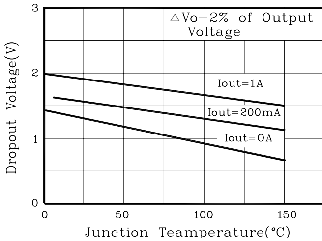
Fig. 1 V_{DVSE} T_j
