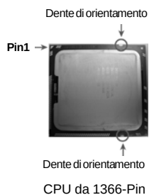
CPU da 1366-Pin
