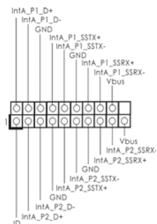
USB 3.0 擴充接頭 (19 針 USB3_L2) (見第 2 頁第 23 項)
