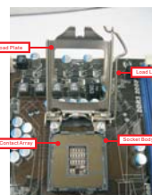
Vista del socket 1155-Pin
