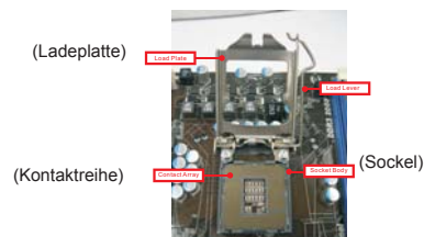
1155-Pin Sockel Übersicht
