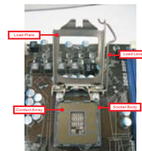
1155 ピンソケットの概要
