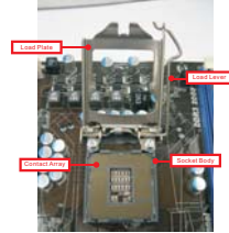
1155-Pinli Sokete Genel Bakış
