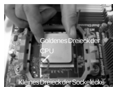
SCHRITT 2 / SCHRITT 3: Richten Sie das goldene Dreieck der CPU mit dem kleinen Dreieck der Sockellecke aus
