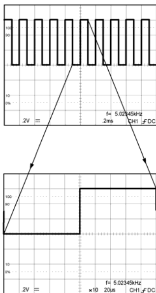
图 5-8 放大的波形
