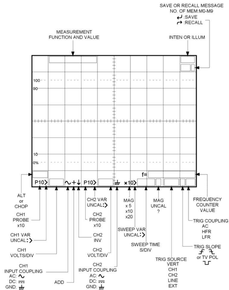
图 5-1 读出版面
