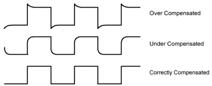
图 5-2 典型的补偿波形
