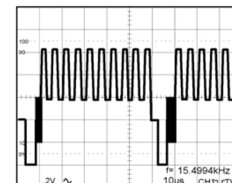
图 5-14(b) TV-H
