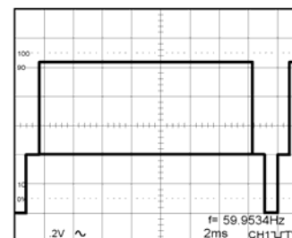
图 5-14(a) TV-V
