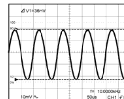
图 5-16 光标测量
