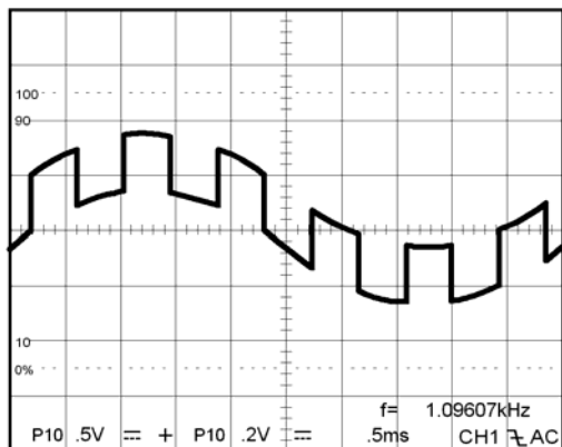
图 5-6 典型 ADD 波形
