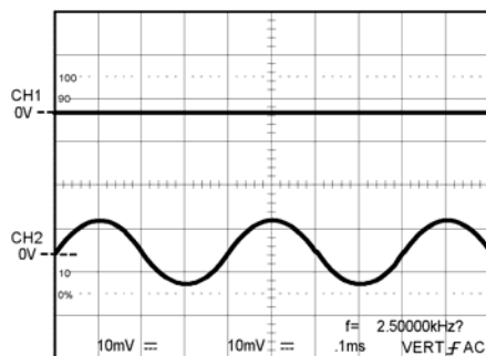
图 5-12 VERT 模式下一通道触发源
