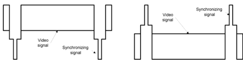
图 5-15 TV 信号
