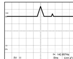
图 5-9(a) MAG x1 波形
