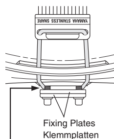
Position the loop between these Die Schlaufe dazwischenlegen
