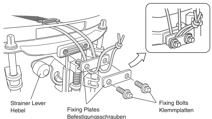
[Abbildung 2] Abhebemechanismus
