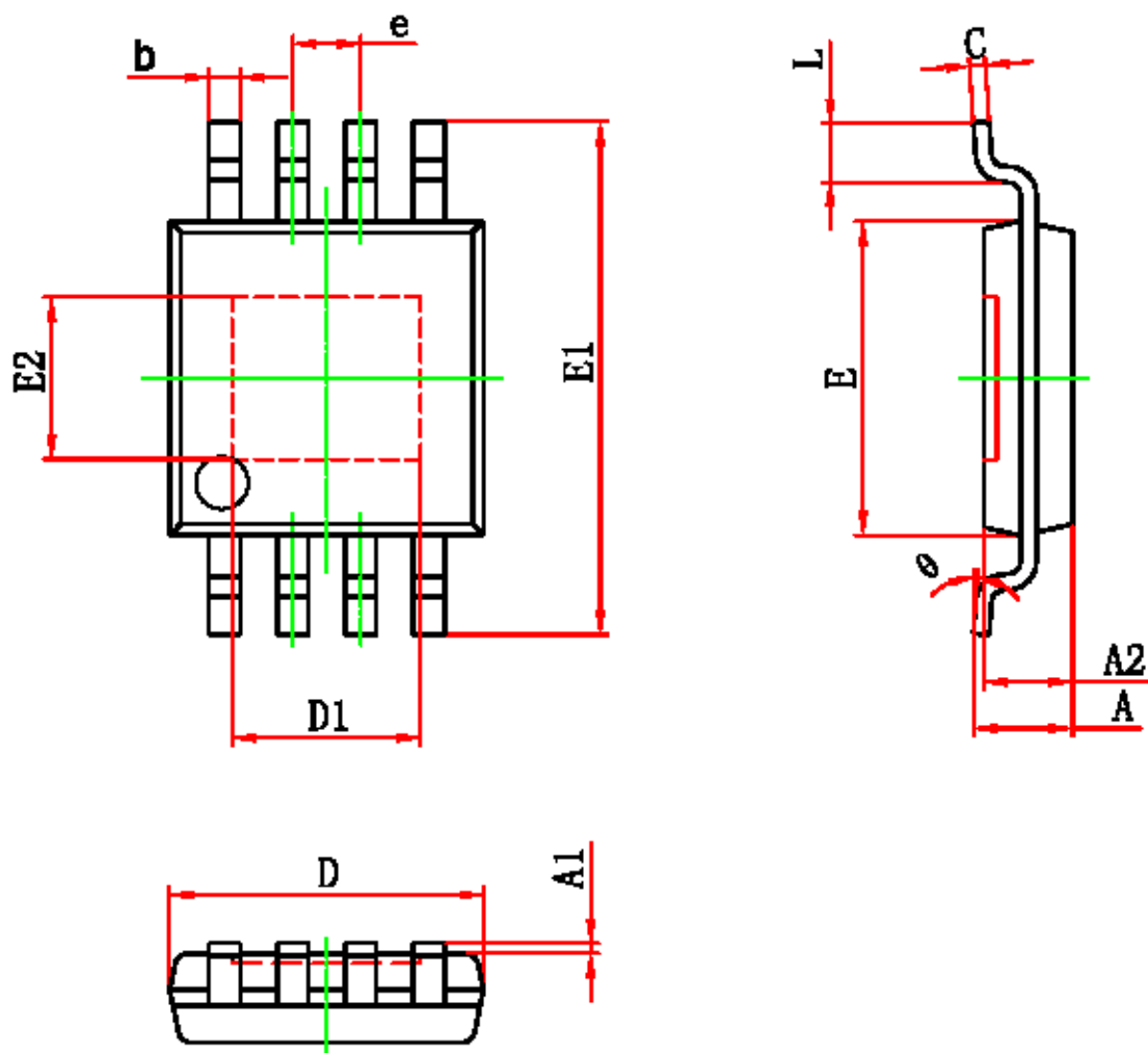
8 引脚 MSOP-PP 封装 (单位 mm)
