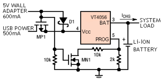
图 6: 交流适配器与 USB 电源的组合
