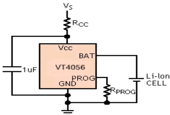
图 3：一种尽量增大热调节模式充电电流的电路
