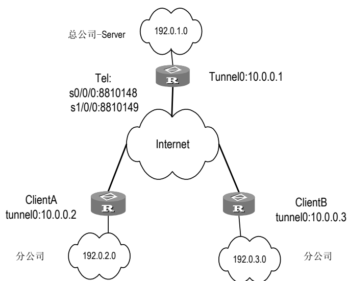
图4-3 Client 通过拨号方式连接 DVPN Server 配置举例
