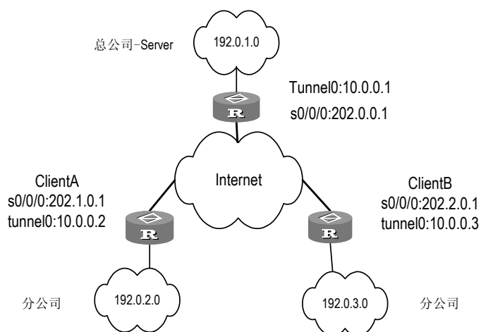
图4-2 动态VPN典型配置应用
