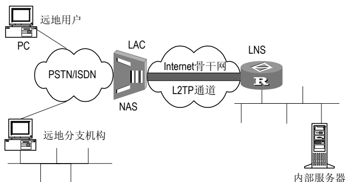
图2-1 应用 L2TP 构建的 VPDN 服务
