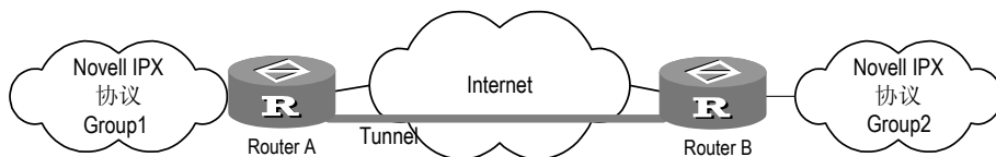
图3-1 IPX 网络通过 GRE 隧道互连
