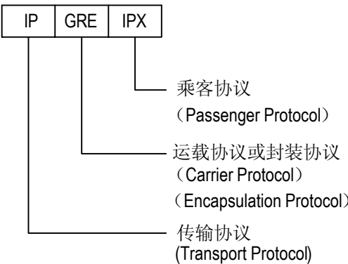
图3-3 Tunnel 中传输报文的格式
