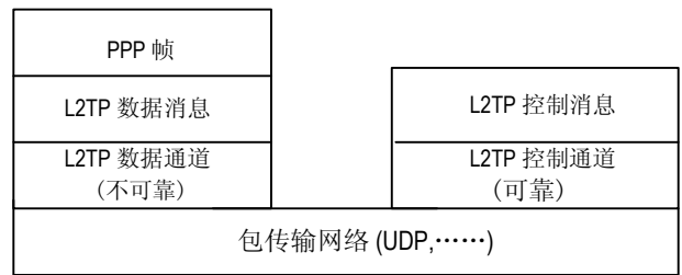
图2-2 L2TP 协议结构
