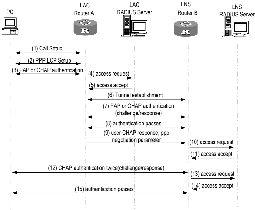
图2-5 L2TP 隧道的呼叫建立流程
