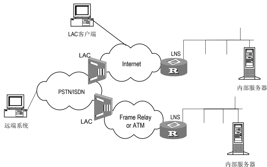
图2-3 两种典型的 L2TP 隧道模式
