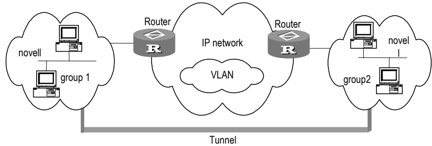
图3-6 Tunnel 连接不连续子网
