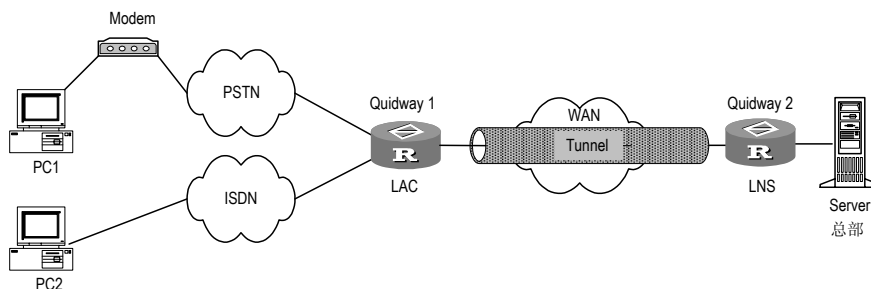
图2-8 单用户与总部互联示意图
