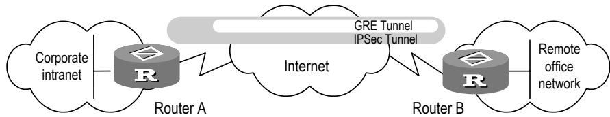
图3-7 GRE-IPSec 隧道应用
