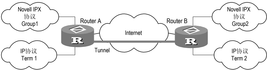
图3-4 多协议本地网通过单一协议骨干网传输
