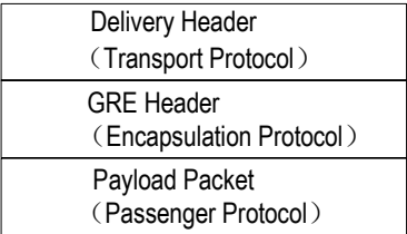
图3-2 封装好的 Tunnel 报文格式
