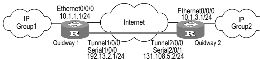
图3-8 GRE 应用组网图
