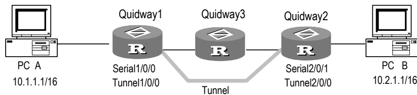
图3-9 GRE 排错示例
