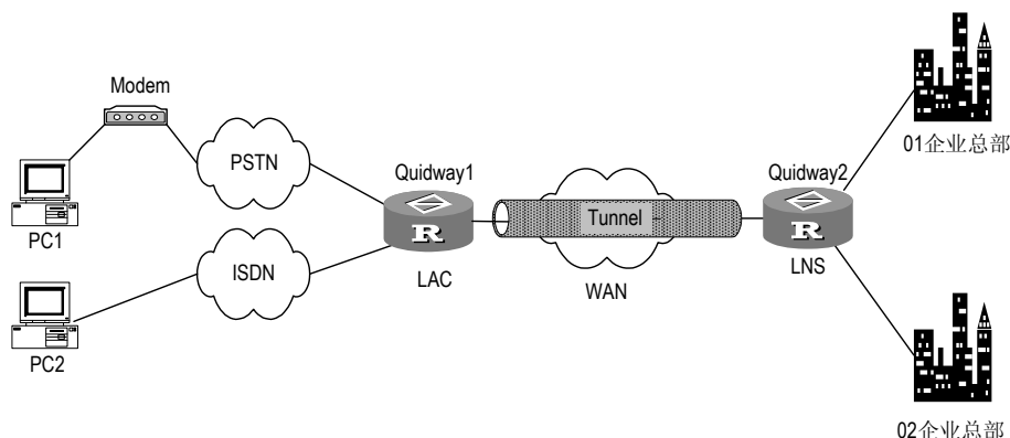
图2-9 L2TP 支持多实例组网图
