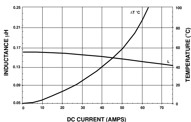
IHLP-5050CE-01 0.15 \mu H
