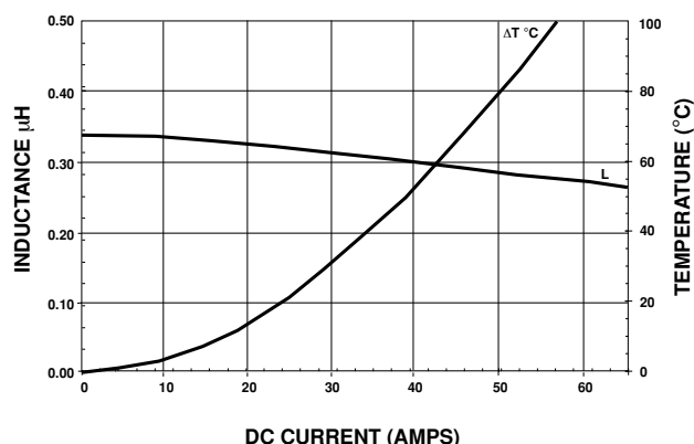
IHLP-5050CE-01 0.33 \mu H
