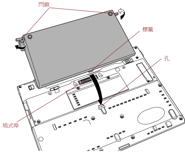
圖 6-3 薄型擴充電池就位
