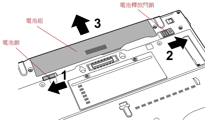
圖 6-1 釋放電池組
