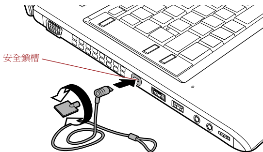
圖 3-15 安全鎖
