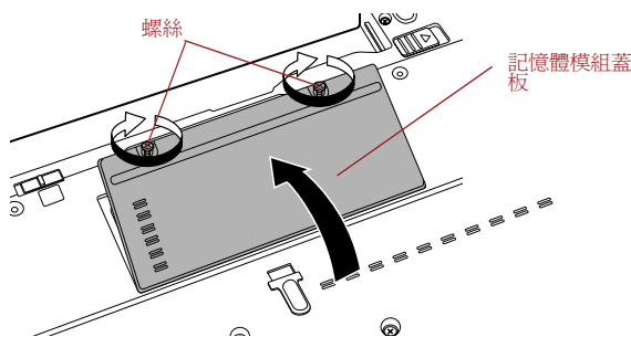
圖 3-9 記憶體模組蓋板就位
