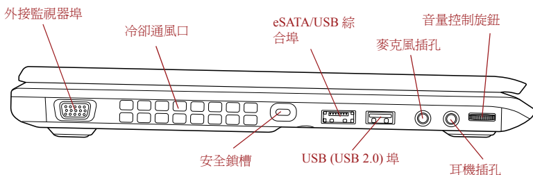
圖 2-2 電腦的左側
