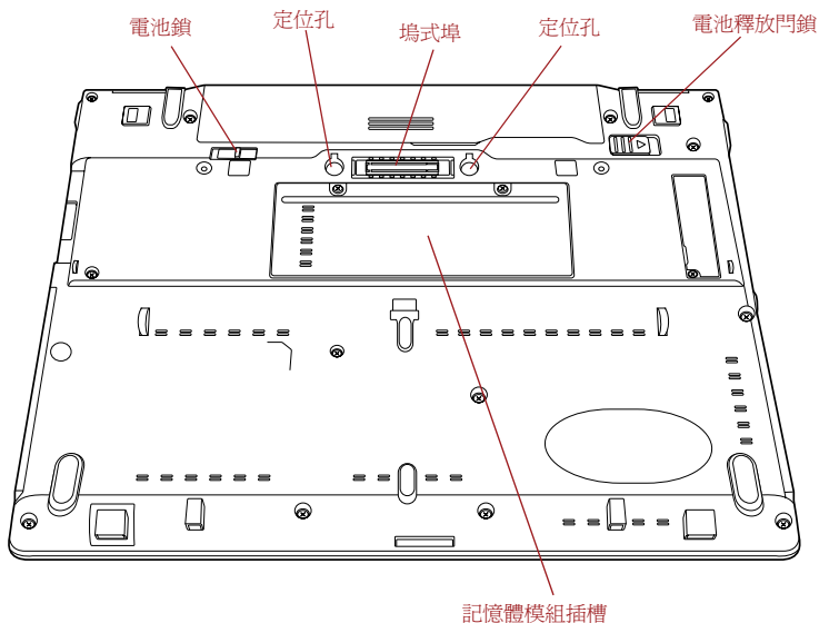
圖 2-5 電腦的底部
