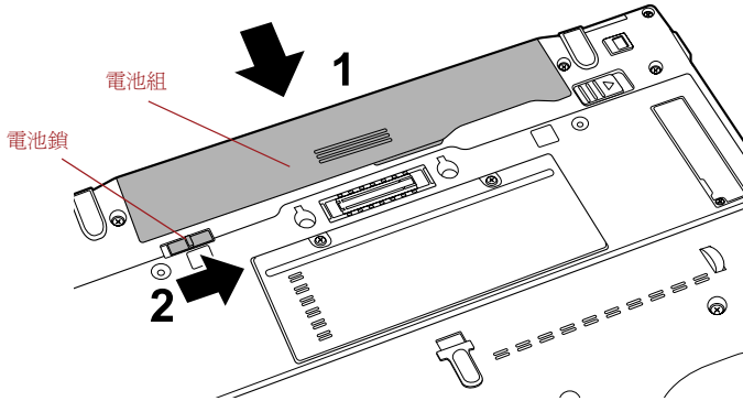
圖 6-2 固定電池組
