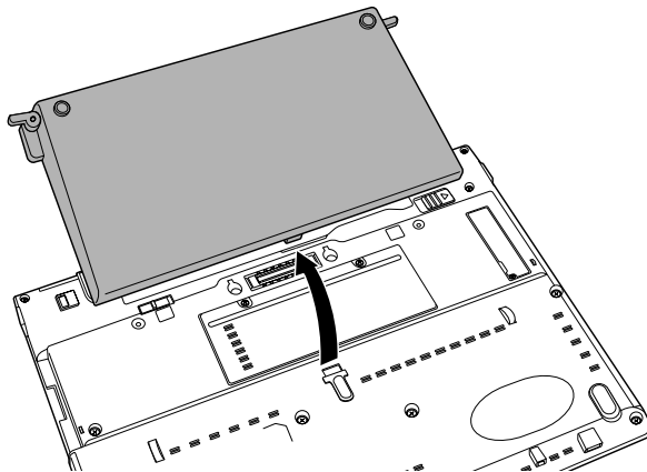
圖 6-6 移除薄型擴充電池
