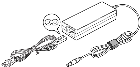
圖 2-10 AC 變壓器 (2 腳插頭)
