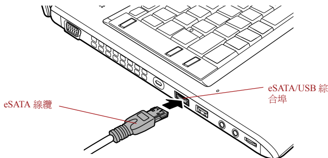
圖 3-14 將 eSATA 線纜連線至 eSATA/USB 綜合埠
