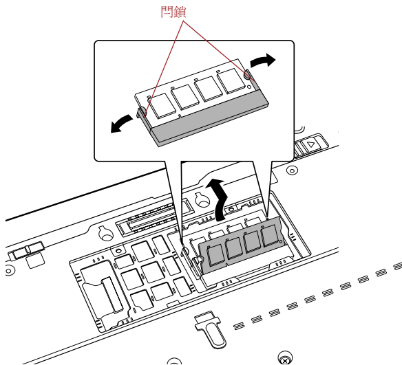
圖 3-10 移除記憶體模組
