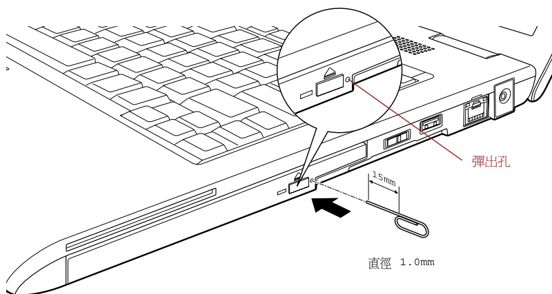
圖 4-8 使用彈出孔手動釋放托架
