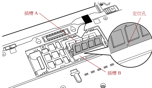
圖 3-8 記憶體模組就位
