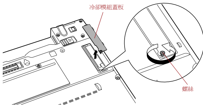
圖 G-1 移除冷卻模組蓋板
