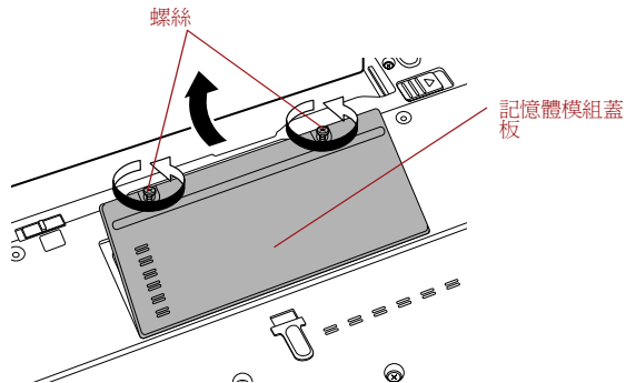
圖 3-7 移除記憶體模組蓋板
