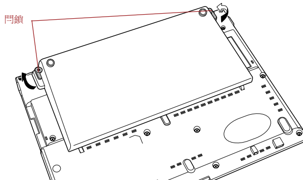
圖 6-5 釋放門鎖
