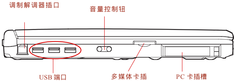
图 2-2 电脑的左侧面板部件示意图
