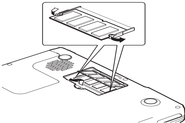
图 8-7 移除内存模块示意图
