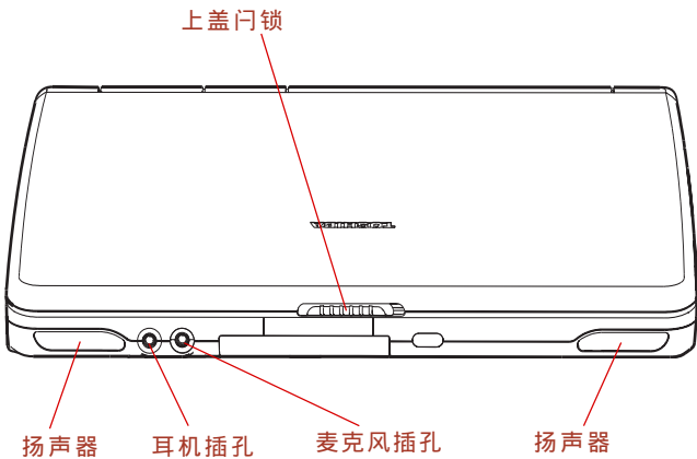
图 2-1 当电脑的显示屏合上时的前面板部件示意图
