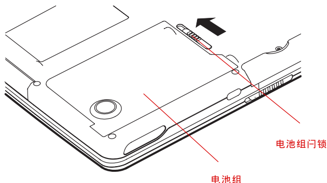
图 6-1 推动电池门锁
