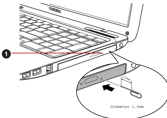
1. Eject hole
